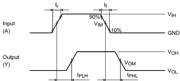
図 11.6.1 t_{PLH} , t_{PHL}
