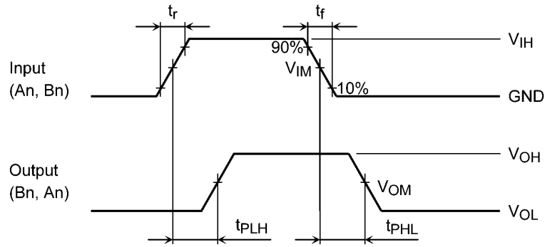
図 11.6.1 tPLH, tPHL
