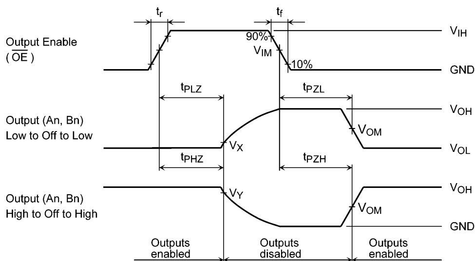
图 11.6.2 t_{PLZ} , t_{PHZ} , t_{PZL} , t_{PZH}
