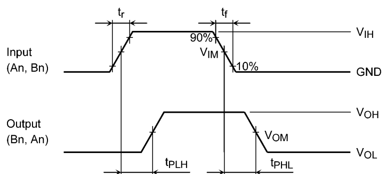
图 11.6.1 t_{PLH} , t_{PHL}
