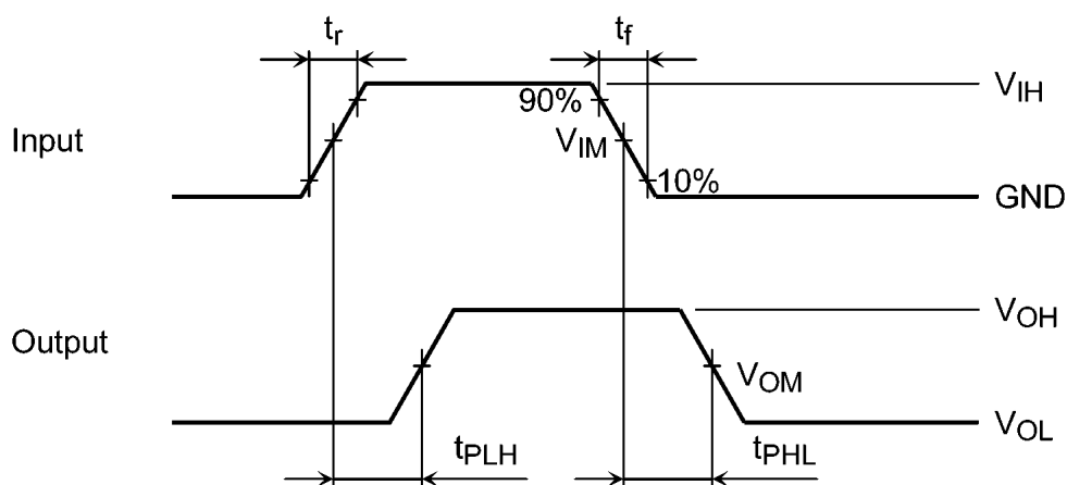
図 11.8.1 t_{PLH} , t_{PHL}
