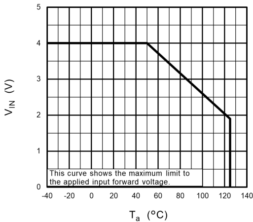
Fig. 12.1 V_{IN} - T_a
