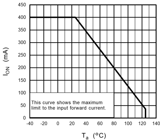
Fig. 12.3 I_{ON} - T_a
