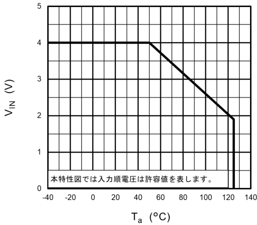
図 12.1 V_{IN} - T_a
