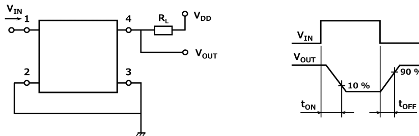
図 11.1 スwitching時間測定回路, 波形
