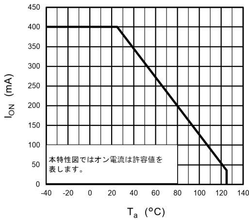
図 12.3 I_{ON} - T_a
