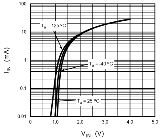
図 12.2 I_{IN} - V_{IN}
