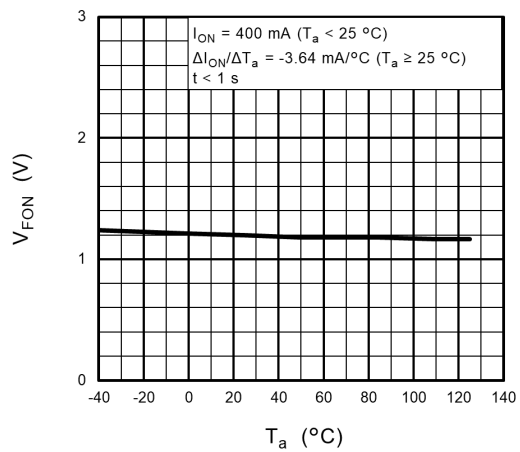
図 12.6 V_{FON} - T_a
