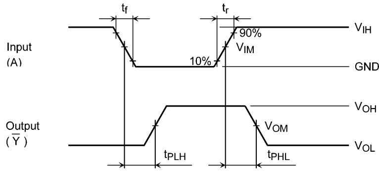
図 11.6.1 tPLH, tPHL
