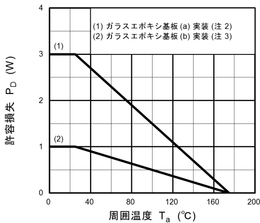
図 8.15 P_D - T_a (最大値 (保証値))
