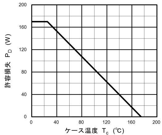
図 8.16 P_D - T_c (Bottom drain) (最大値 (保証値))
