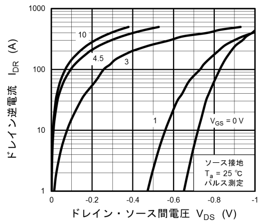
図 8.6 I_{DR} - V_{DS}
