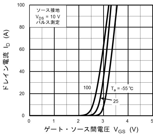
図 8.3 I_D - V_{GS}
