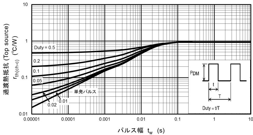
図 8.14 r_{th} - t_w (Top source) (最大値 (保証値))
