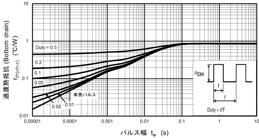
図 8.13 r_{th} - t_w (Bottom drain) (最大値 (保証値))
