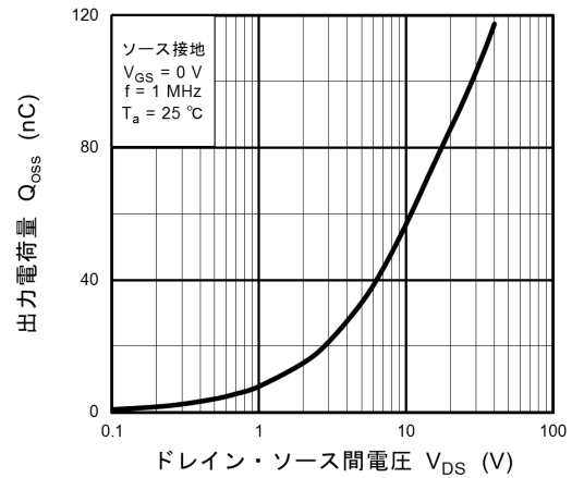
図 8.12 Q_{oss} - V_{DS}
