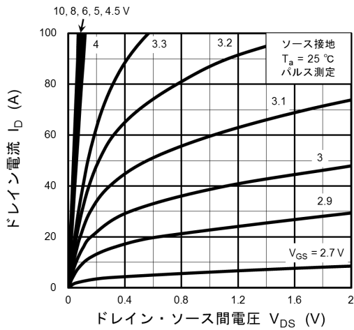
図 8.1 I_D - V_{DS}
