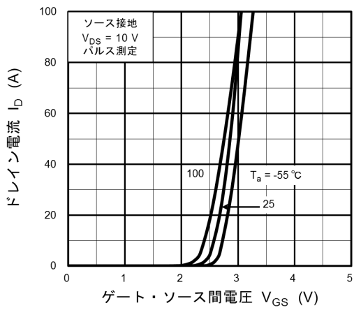
図 8.3 I_D - V_{GS}
