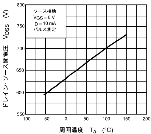
図 8.5 V_{DS} - T_a
