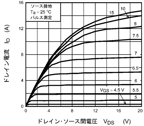
図 8.2 I_D - V_{DS}
