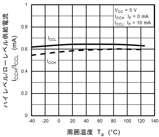
図 13.2.11 I_{CCH}, I_{CCL} - T_a
