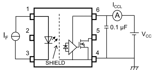
図 13.1.4 I CCL 測定回路
