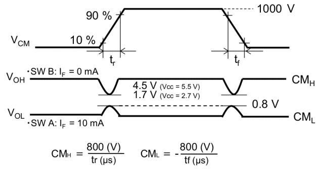
図 13.1.7 コモンモードノイズ除去電圧測定回路, 波形
