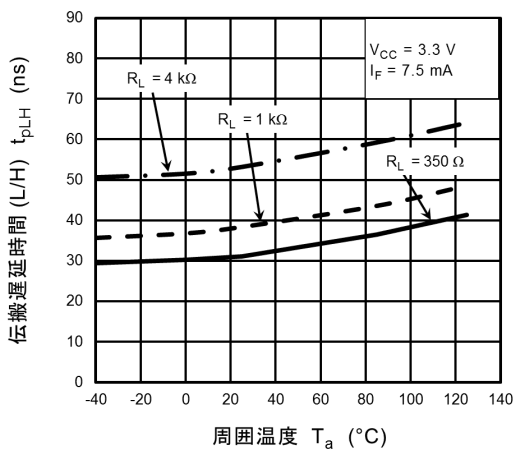
図 13.2.17 t_{pLH} - T_a
