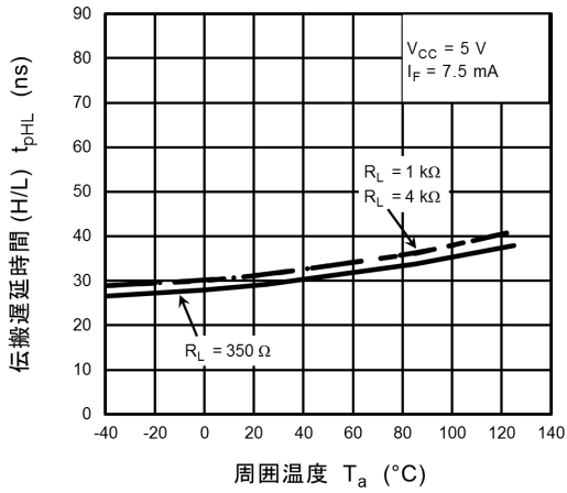
図 13.2.13 t_{pHL} - T_a
