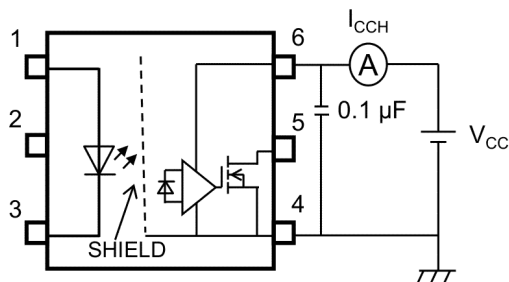
図 13.1.3 I_{CCH} 測定回路
