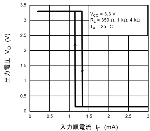
図 13.2.6 V_O - I_F
