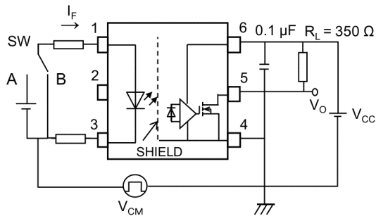
図 13.1.7 コモンモードノイズ除去電圧測定回路, 波形
