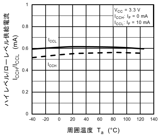
図 13.2.12 I_{CCH}, I_{CCL} - T_a
