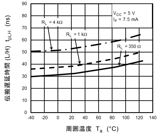
図 13.2.14 t_{pLH} - T_a
