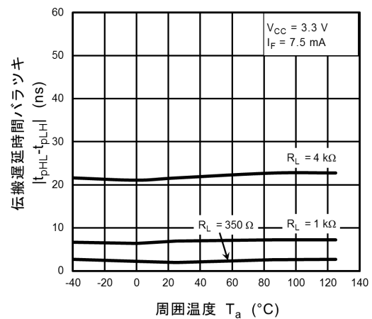
図 13.2.18 |t_{pHL} - t_{pLH}| - T_a
