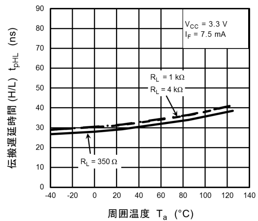
図 13.2.16 t_{pHL} - T_a
