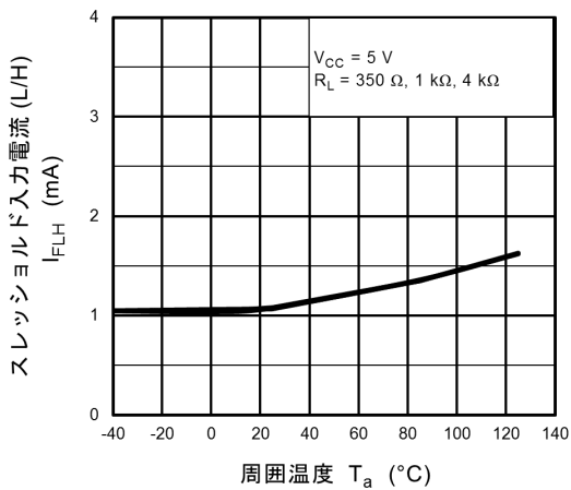
図 13.2.9 I_{FLH} - T_a
