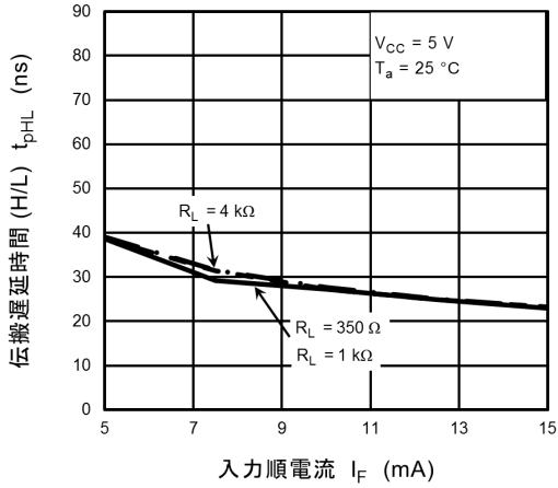
図 13.2.19 t_{pHL} - I_F
