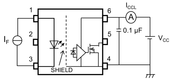
図 13.1.4 I_{CCL} 測定回路
