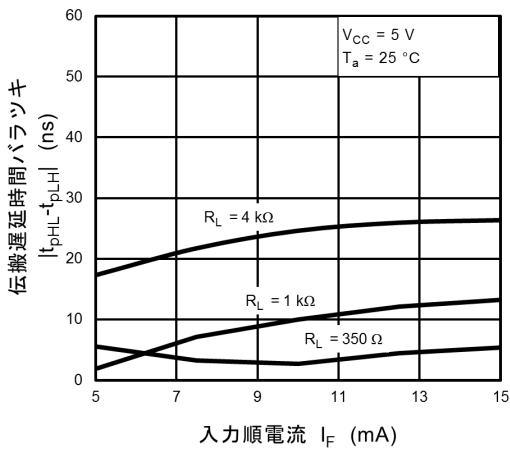
図 13.2.21 |t_{pHL} - t_{pLH}| - I_F
