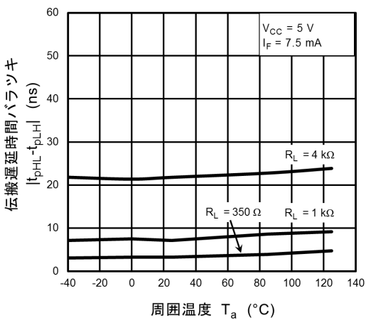
図 13.2.15 |t_{pHL} - t_{pLH}| - T_a
