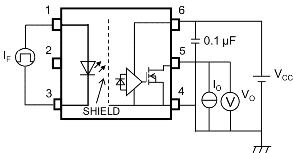
図 13.1.5 I_{FHL} , I_{FLH} , I_{HYS} 測定回路
