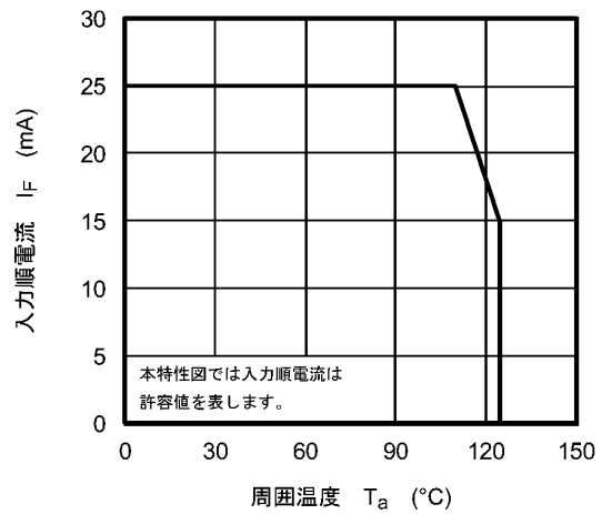
図 13.2.2 I_F - T_a
