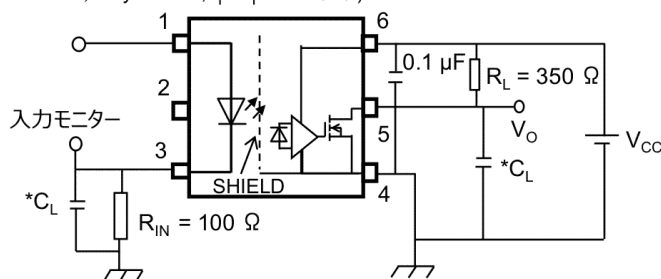
図 13.1.6 伝搬遅延時間測定回路, 波形
