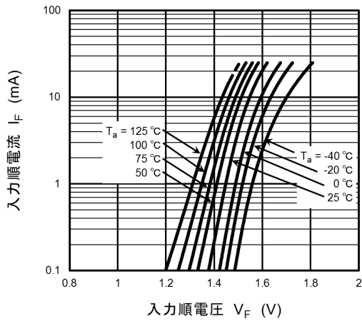
図 13.2.1 I_F - V_F
