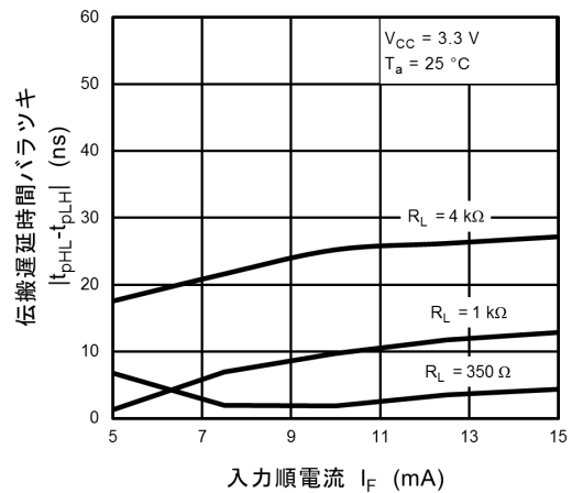
図 13.2.24 |t_{pHL} - t_{pLH}| - I_F
