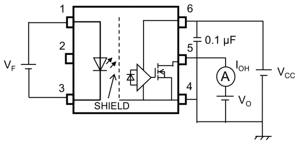
図 13.1.1 I_{OH} 測定回路
