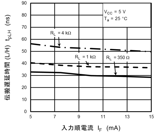
図 13.2.20 t_{pLH} - I_F
