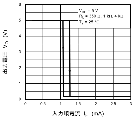
図 13.2.5 V_O - I_F
