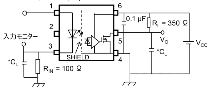
図 13.1.6 伝搬遅延時間測定回路, 波形
