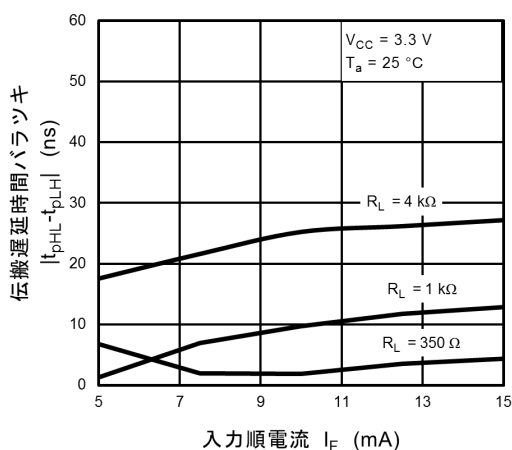
図 13.2.24 |t_{pHL} - t_{pLH}| - I_F
