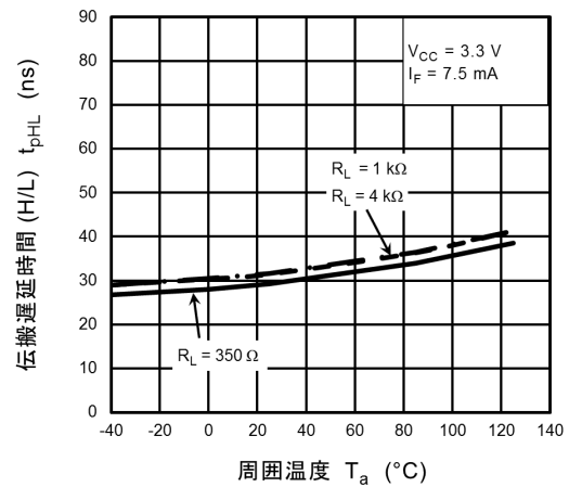
図 13.2.16 t_{pHL} - T_a
