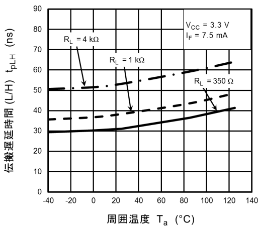
図 13.2.17 t_{pLH} - T_a
