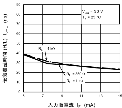
図 13.2.22 t_{pHL} - I_F
