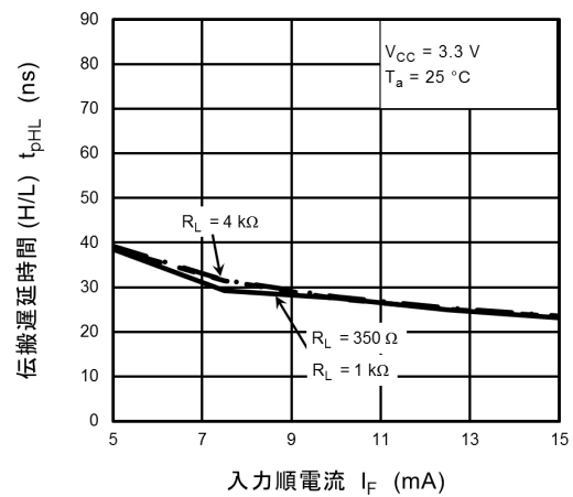
図 13.2.22 t_{pHL} - I_F
