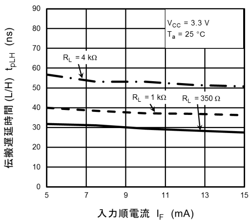
図 13.2.23 t_{pLH} - I_F
