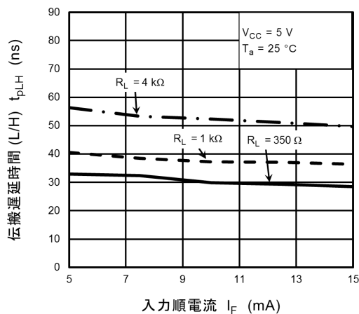
図 13.2.20 t_{pLH} - I_F
