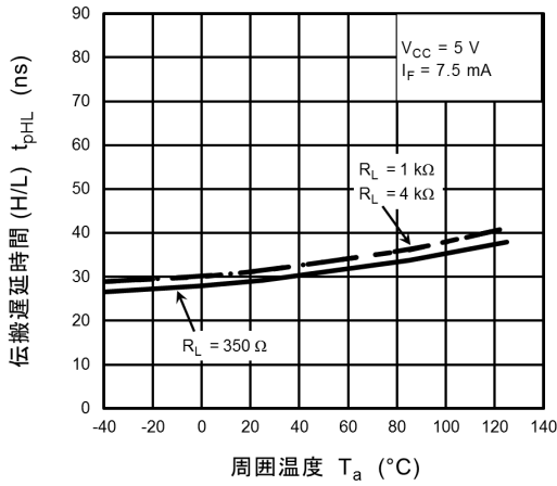
図 13.2.13 t_{pHL} - T_a
