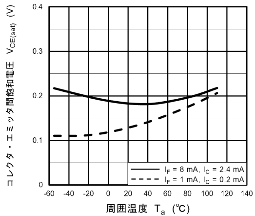
図 11.10 V_{CE(\text{sat})} - T_a
