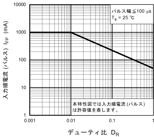
図 11.3 I_{FP} - D_R
