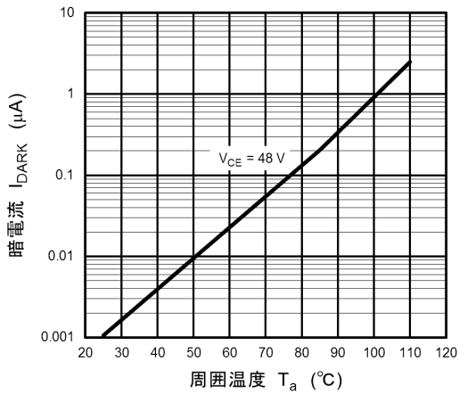
図 11.9 I_{\text{DARK}} - T_a
