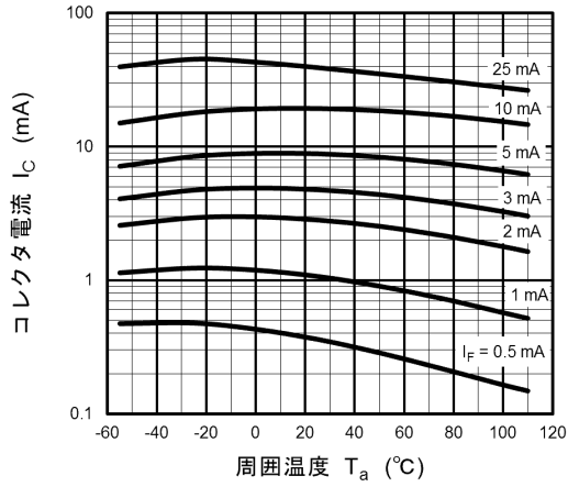
図 11.13 I_C - T_a
