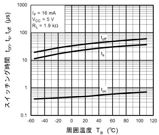
図 11.15 スイッチング時間 - T_a
