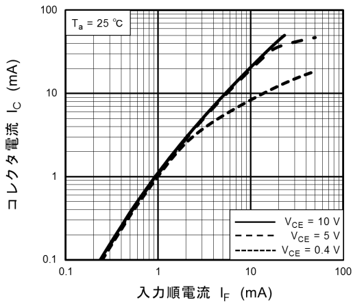
図 11.11 I_C - I_F
