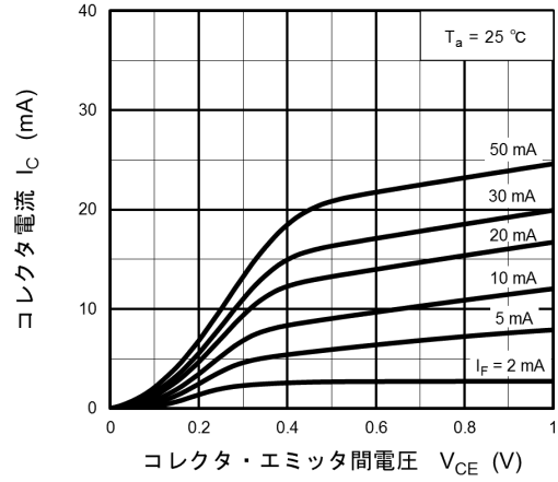
図 11.8 I_C - V_{CE}
