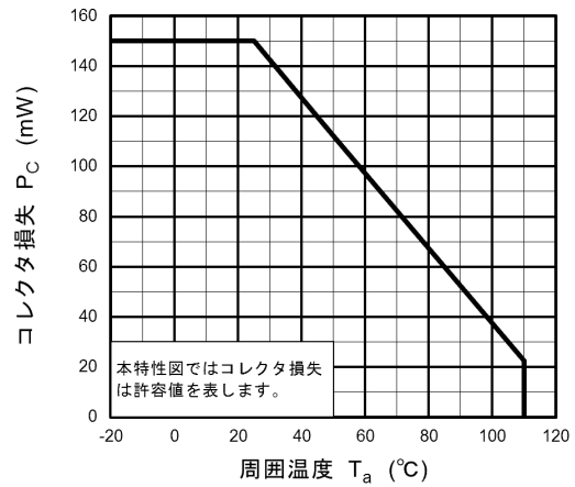
図 11.2 P_C - T_a
