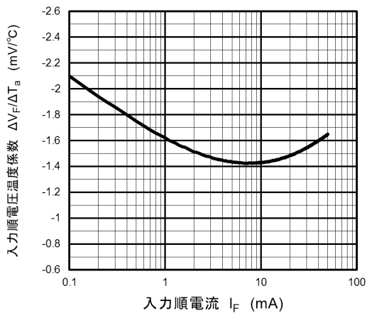
図 11.5 \Delta V_F / \Delta T_a - I_F
