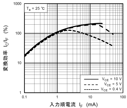
図 11.12 I_C/I_F - I_F
