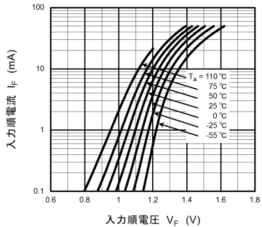
図 11.4 I_F - V_F
