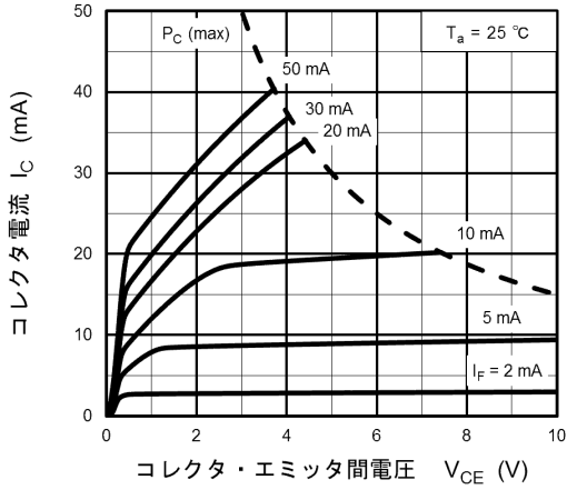
図 11.7 I_C - V_{CE}
