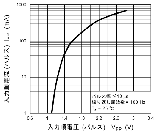
図 11.6 I_{FP} - V_{FP}
