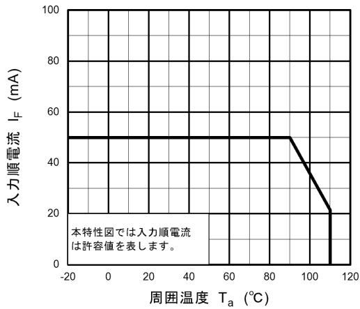
図 11.1 I_F - T_a
