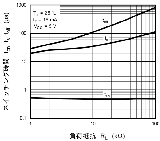
図 11.14 スイッチング時間 - R_L
