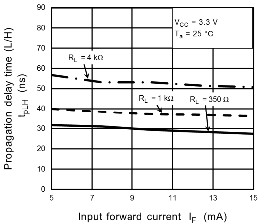
Fig. 13.2.23 t_{pLH} - I_F
