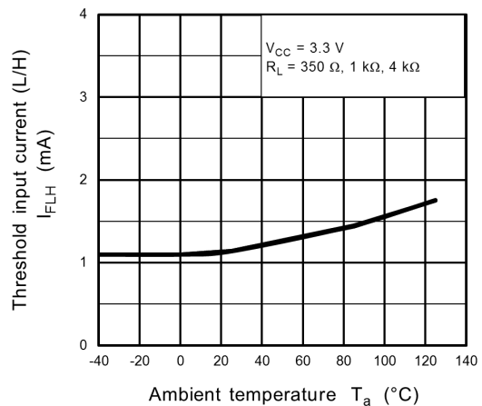
Fig. 13.2.10 I_{FLH} - T_a
