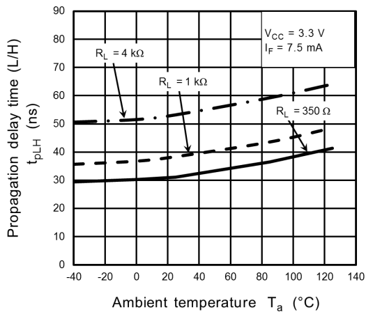
Fig. 13.2.17 t_{pLH} - T_a
