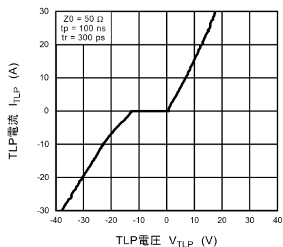
図 10.11.1 I_{TLP} - V_{TLP}
