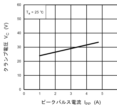
図 10.16.2 V_C - I_{PP}
