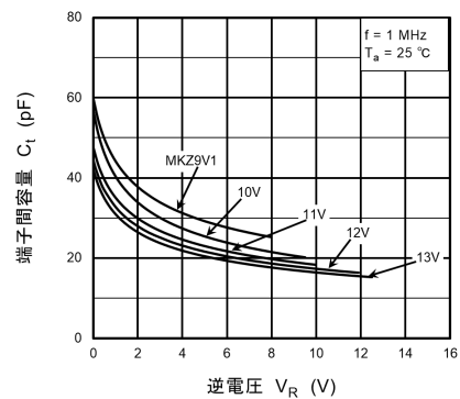
図 10.1.6 C_t - V_R(2)
