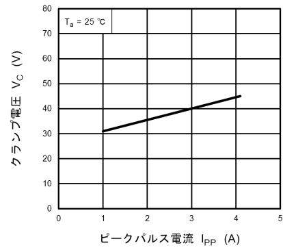
図 10.18.2 V_C - I_{PP}
