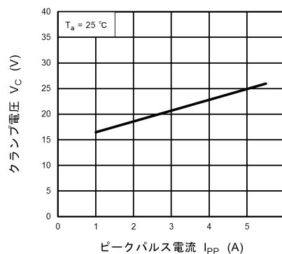
図 10.13.2 V_C - I_{PP}
