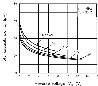
Fig. 10.1.6 C_t - V_R (2)
