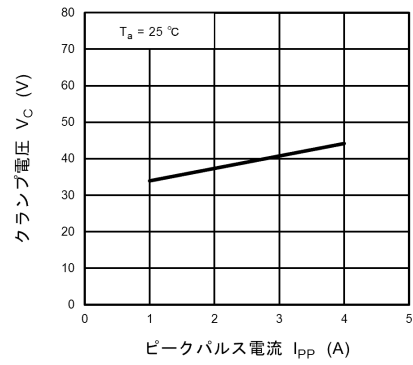
図 10.19.2 V_C - I_{PP}
