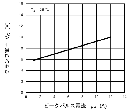
図 10.2.2 V_C - I_{PP}
