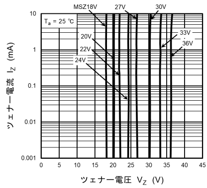
図 10.1.2 I_Z - V_Z(2)
