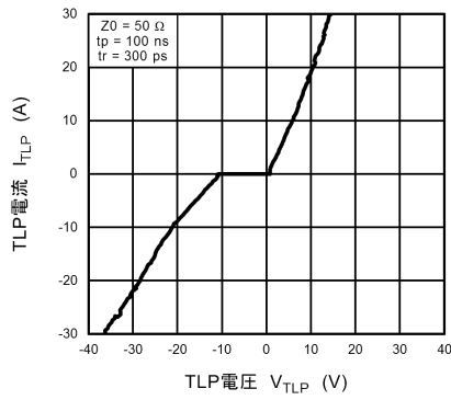
図 10.9.1 I_{TLP} - V_{TLP}
