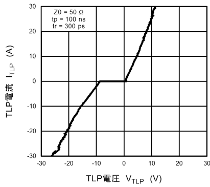
図 10.7.1 I_{TLP} - V_{TLP}
