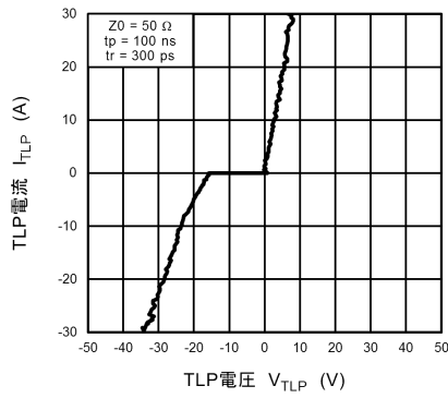
図 10.13.1 I_{TLP} - V_{TLP}
