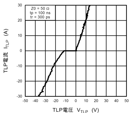
図 10.10.1 I_{TLP} - V_{TLP}
