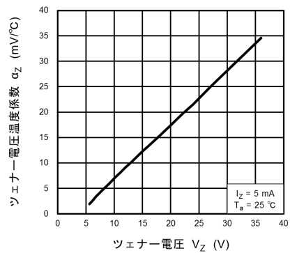
図 10.1.4 \alpha_Z - V_Z
