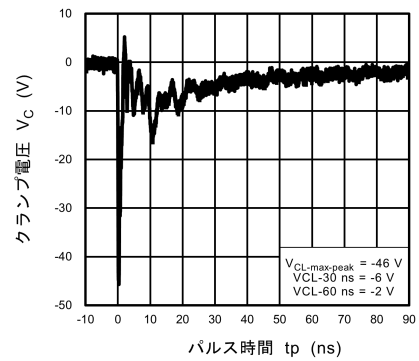
図 10.4.4 IEC61000-4-2 クランプ波形 -8 kV
