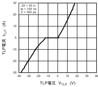
図 10.11.1 I_{TLP} - V_{TLP}
