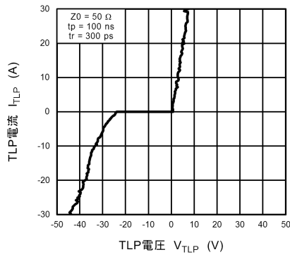
図 10.17.1 I_{TLP} - V_{TLP}
