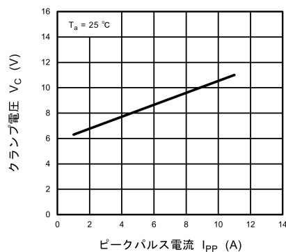
図 10.3.2 V_C - I_{PP}
