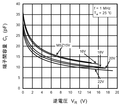
図 10.1.7 C_t - V_R (3)
