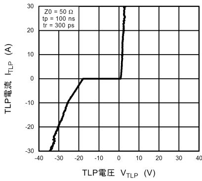
図 10.14.1 I_{TLP} - V_{TLP}
