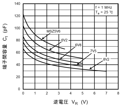
図 10.1.5 C_t - V_R (1)
