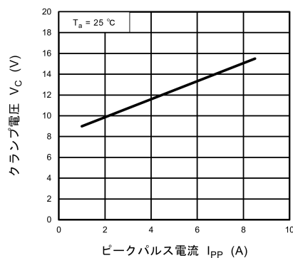
図 10.6.2 V_C - I_{PP}
