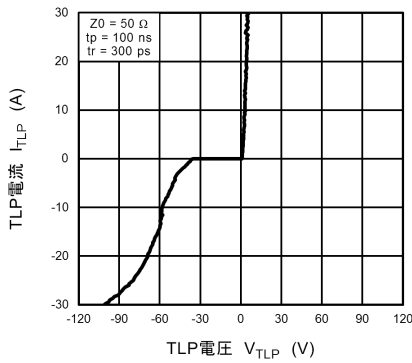
図 10.21.1 I_{TLP} - V_{TLP}
