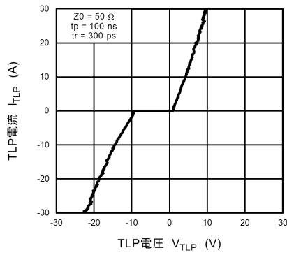
図 10.8.1 I_{TLP} - V_{TLP}
