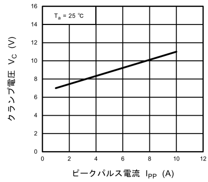
図 10.4.2 V_C - I_{PP}
