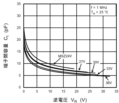
図 10.1.8 C_t - V_R (4)
