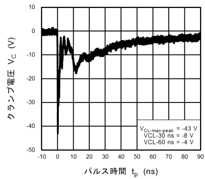
図 10.7.4 IEC61000-4-2 クランプ波形 -8 kV
