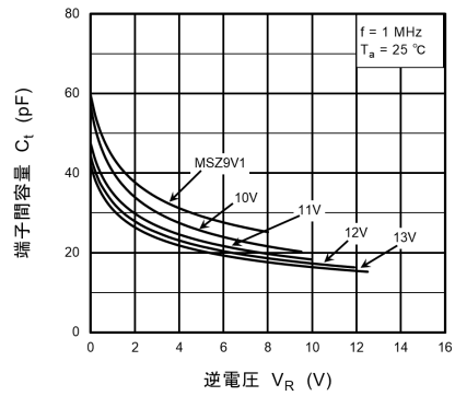
図 10.1.6 C_t - V_R (2)
