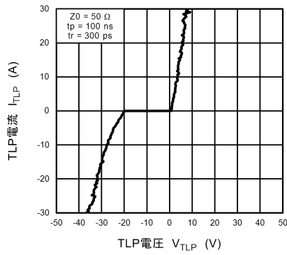
図 10.15.1 I_{TLP} - V_{TLP}
