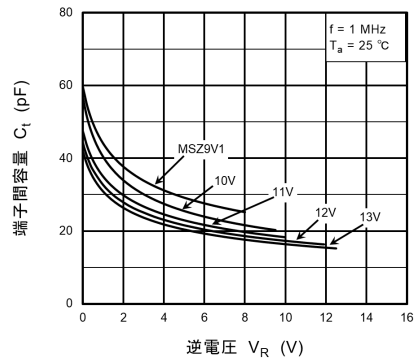
図 10.1.6 C_t - V_R (2)
