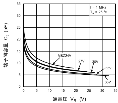
図 10.1.8 C_t - V_R (4)
