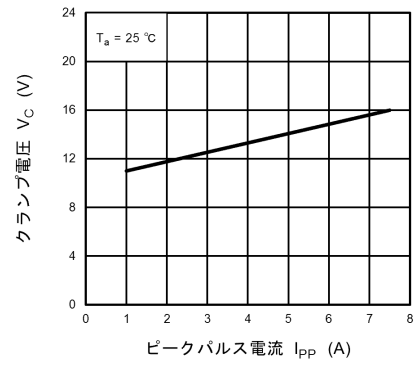
図 10.8.2 V_C - I_{PP}
