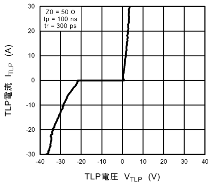
図 10.16.1 I_{TLP} - V_{TLP}
