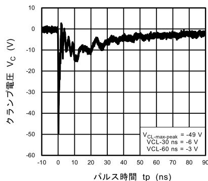
図 10.6.4 IEC61000-4-2 クランプ波形 -8 kV
