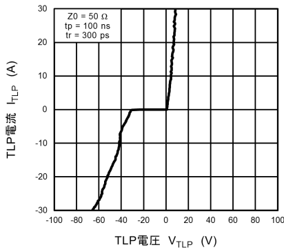
図 10.19.1 I_{TLP} - V_{TLP}
