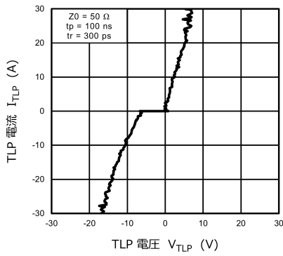
図 10.4.1 I_{TLP} - V_{TLP}
