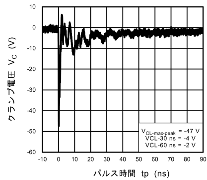
図 10.2.4 IEC61000-4-2 クランプ波形 -8 kV
