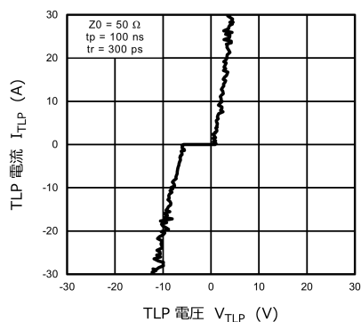
図 10.2.1 I_{TLP} - V_{TLP}
