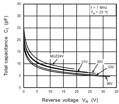
Fig. 10.1.8 C_t - V_R (4)
