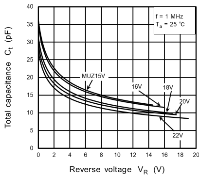
Fig. 10.1.7 C_t - V_R (3)
