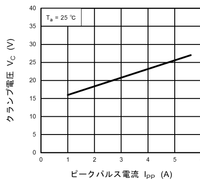
図 10.12.2 V_C - I_{PP}
