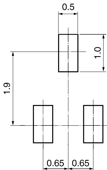
図 9.1 参考パッド寸法(Unit: mm)
