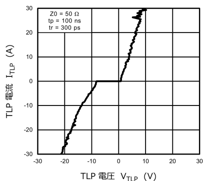
図 10.6.1 I_{TLP} - V_{TLP}
