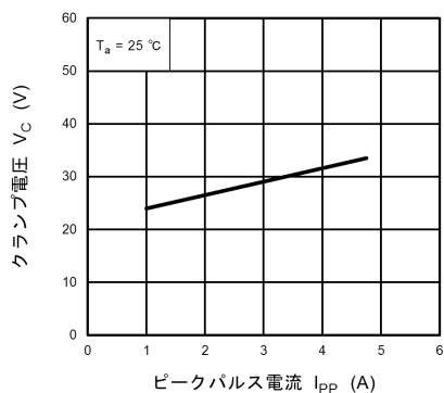
図 10.16.2 V_C - I_{PP}
