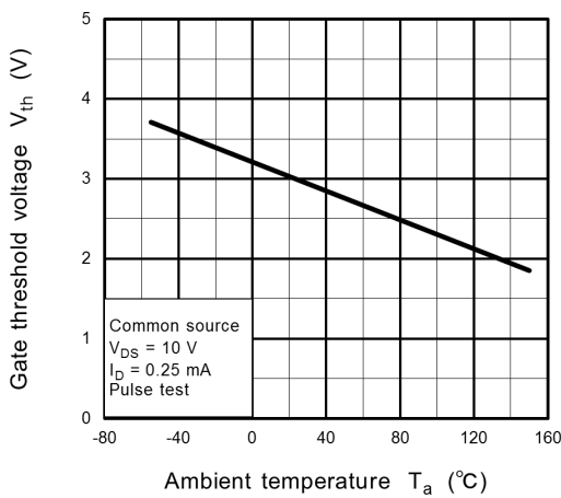
Fig. 8.11 V_{th} - T_a
