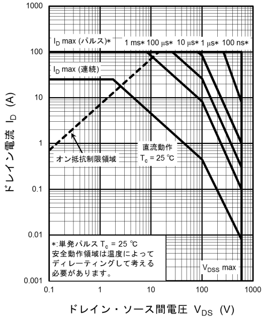
図 8.17 安全動作領域 (最大値 (保証値))
