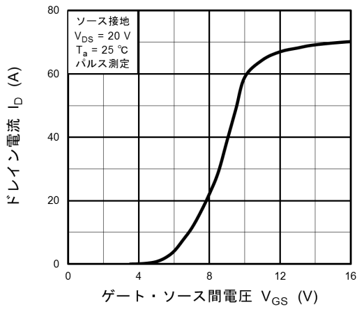
図 8.3 I_D - V_{GS}
