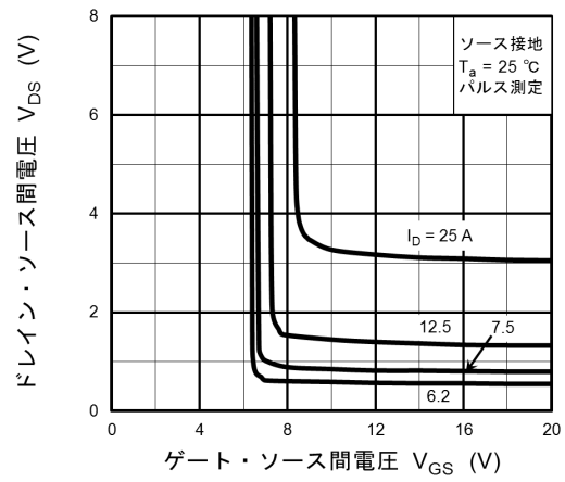
図 8.4 V_{DS} - V_{GS}
