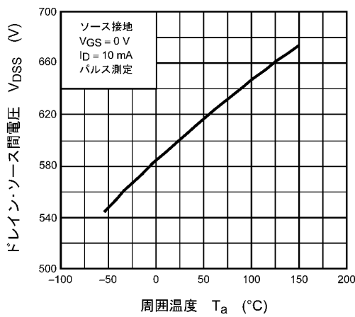
図 8.5 V_{DS} - T_a
