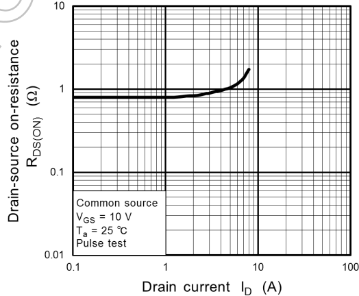
Fig. 8.6 R_{DS(ON)} - I_D
