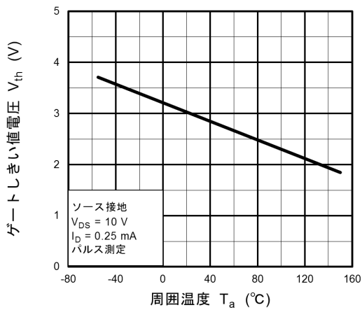
図 8.11 V_{th} - T_a
