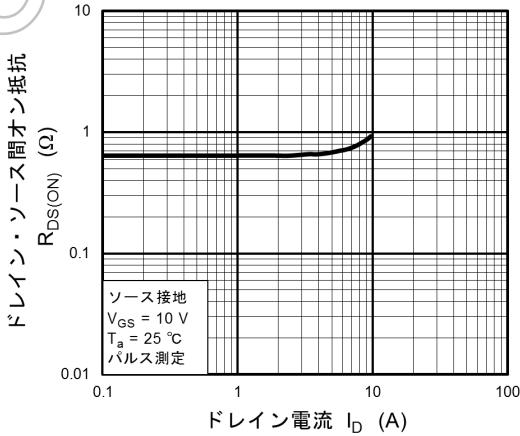
図 8.6 R_{DS(ON)} - I_D
