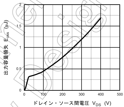
図 8.10 E_{oss} - V_{DS}
