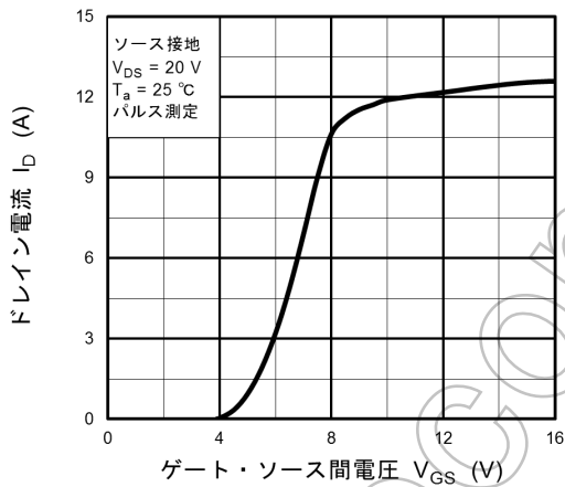
図 8.3 I_D - V_{GS}
