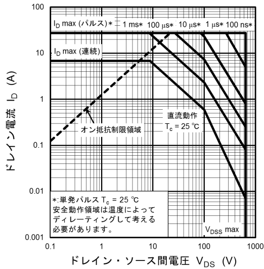
図 8.17 安全動作領域 (最大値 (保証値))
