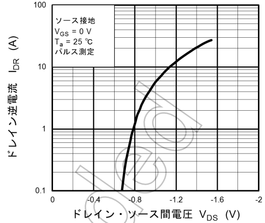
図 8.8 I_{DR} - V_{DS}
