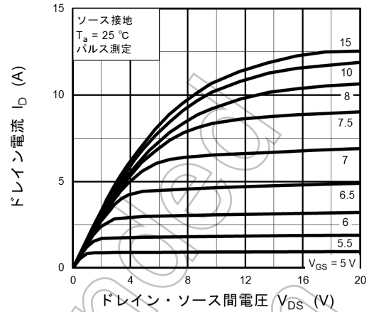
図 8.2 I_D - V_{DS}
