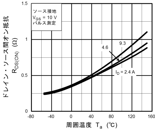
図 8.7 R_{DS(ON)} - T_a
