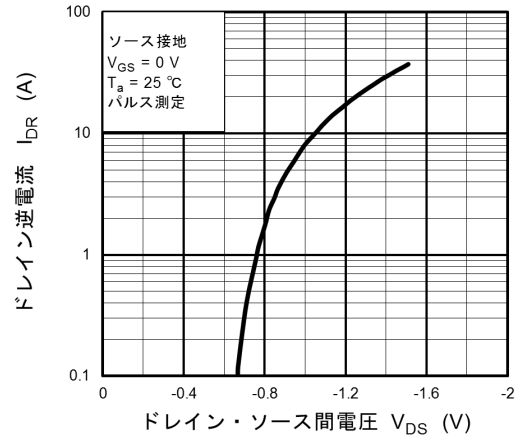
図 8.8 I_{DR} - V_{DS}
