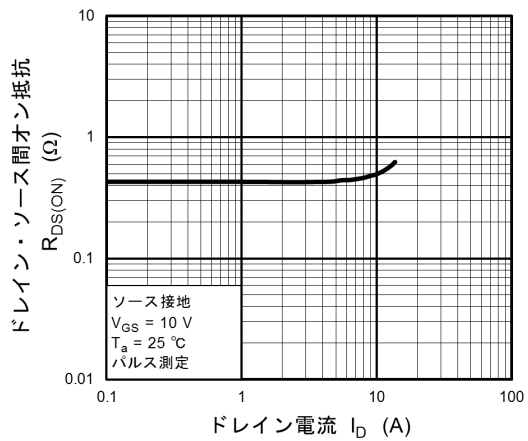
図 8.6 R_{DS(ON)} - I_D
