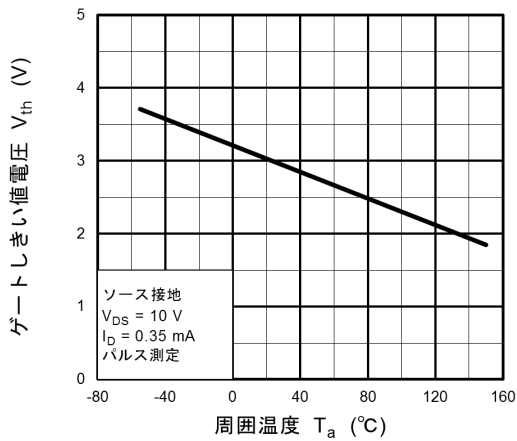
図 8.11 V_{th} - T_a
