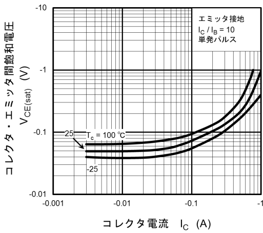
図 7.3 V_{CE(sat)} - I_C
