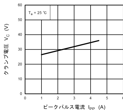
図 10.17.2 V_C - I_{PP}
