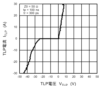
図 10.17.1 I_{TLP} - V_{TLP}
