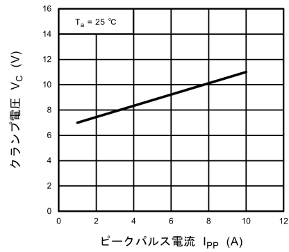
図 10.4.2 V_C - I_{PP}
