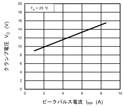
図 10.6.2 V_C - I_{PP}
