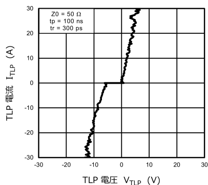
図 10.3.1 I_{TLP} - V_{TLP}
