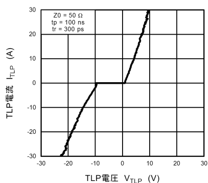
図 10.8.1 I_{TLP} - V_{TLP}
