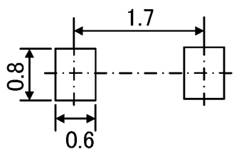
図 9.1 参考パッド寸法(Unit: mm)
