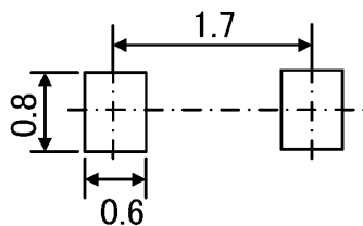
図 9.1 参考パッド寸法(Unit: mm)
