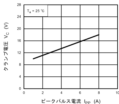
図 10.7.2 V_C - I_{PP}
