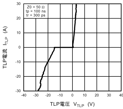
図 10.12.1 I_{TLP} - V_{TLP}
