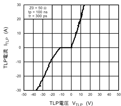
図 10.10.1 I_{TLP} - V_{TLP}
