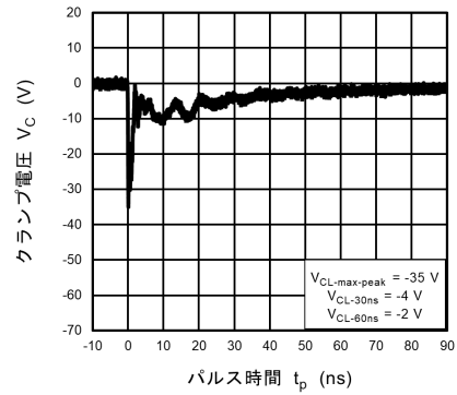
図 10.20.4 IEC61000-4-2 クランプ波形 -8 kV
