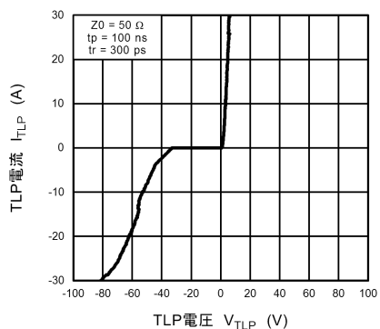
図 10.20.1 I_{TLP} - V_{TLP}
