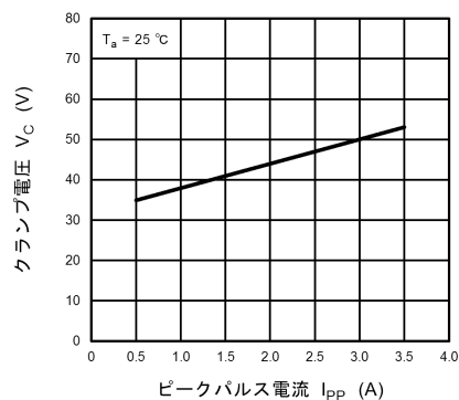
図 10.20.2 V_C - I_{PP}
