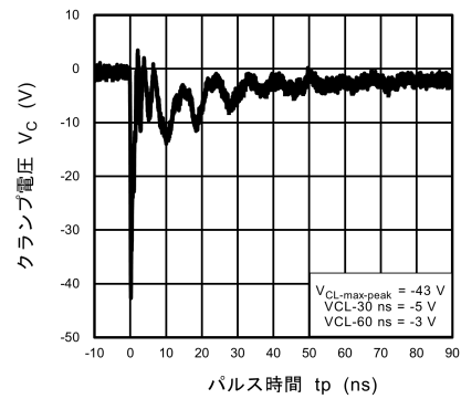
図 10.3.4 IEC61000-4-2 クランプ波形 -8 kV
