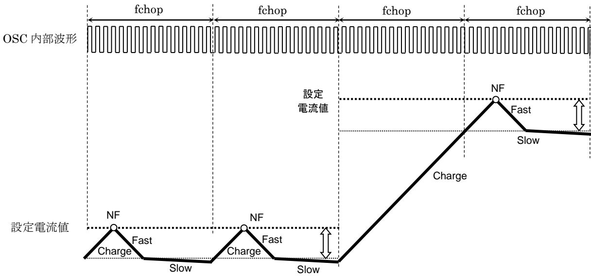
図 6.12 Charge 期間が fchop 1 周期以上の場合
