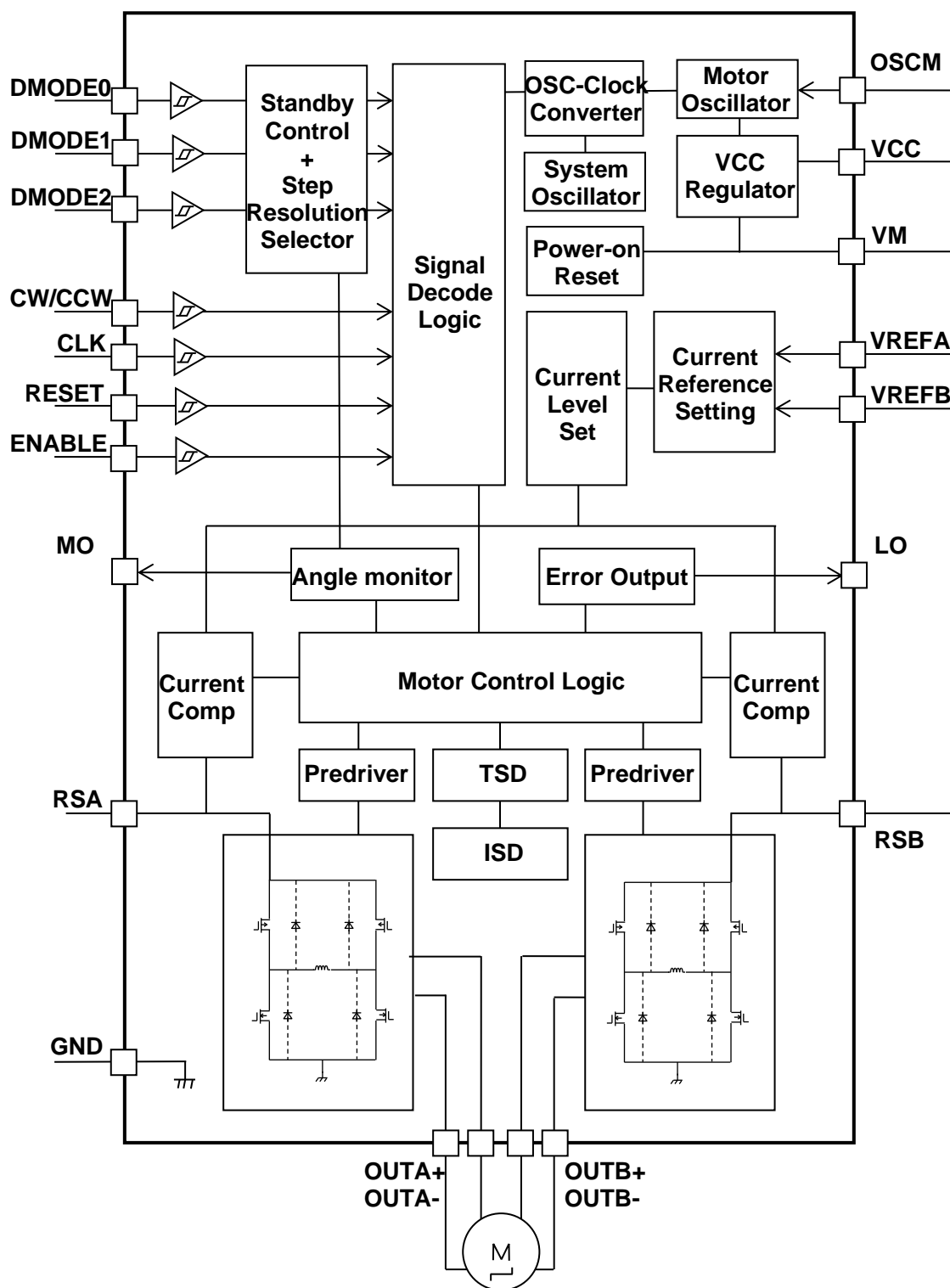
図 3.1 ブロック図
