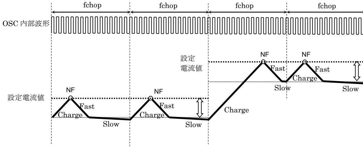
図 6.11 設定電流値が増加方向の場合
