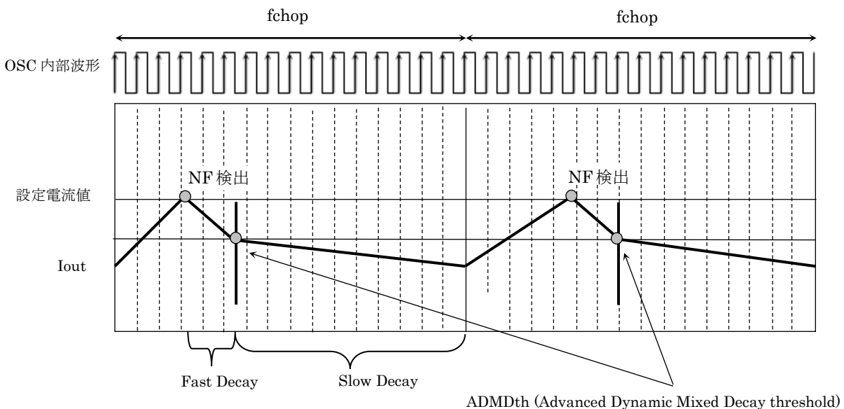
図 6.10 Auto Decay Mode の波形(電流波形)
