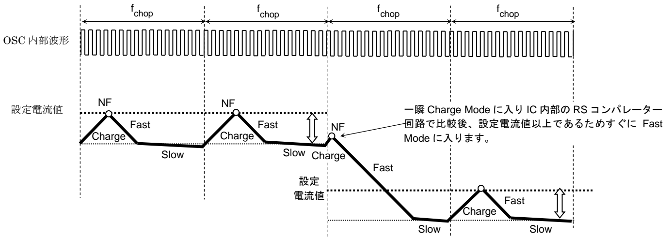
図 6.13 設定電流値が減少方向の場合
