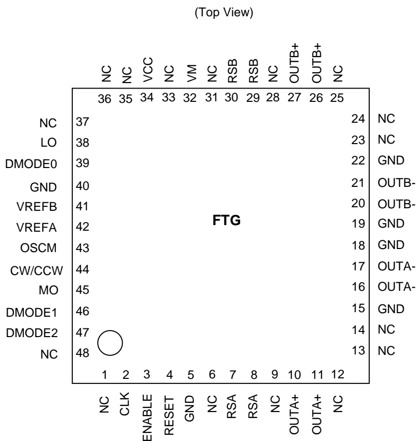
図 4.1 端子配置図
