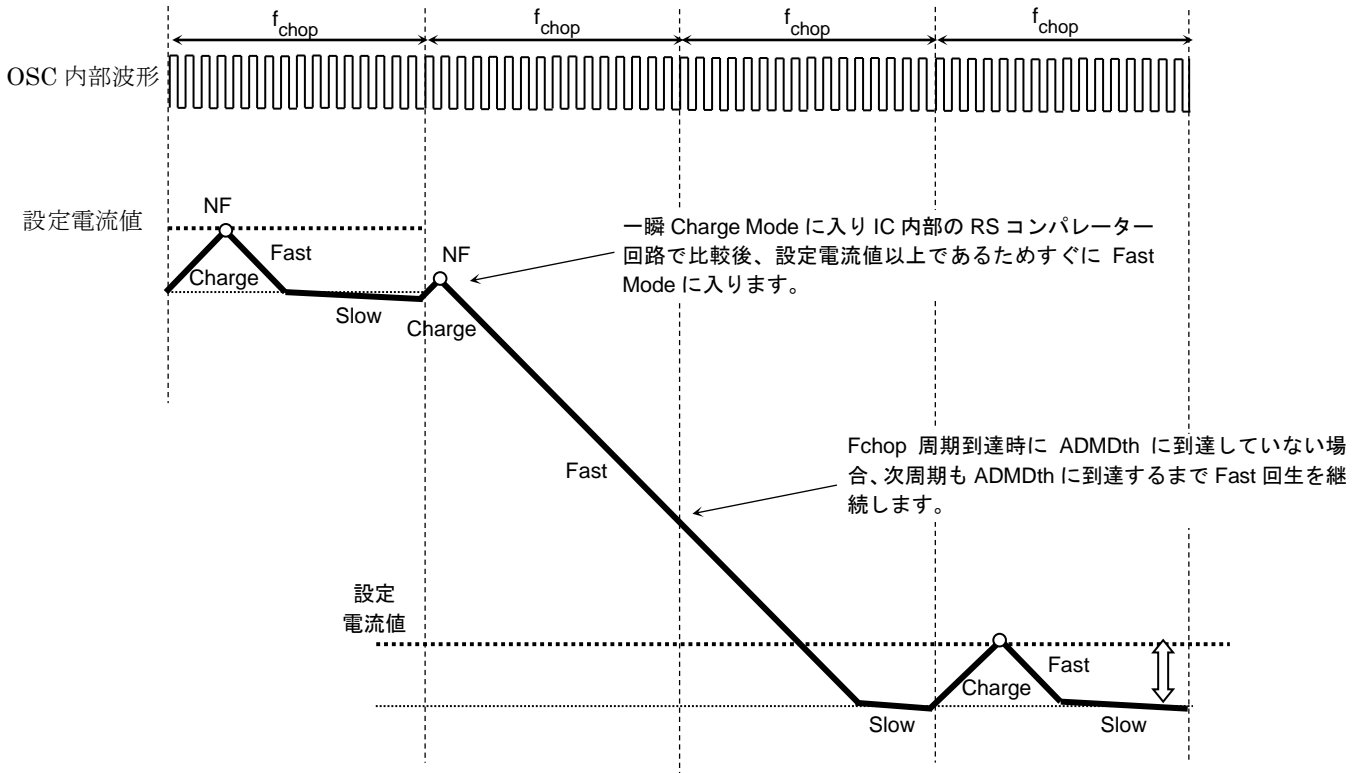
図 6.14 Fast 期間中に f_chop 1 周期到達する場合
