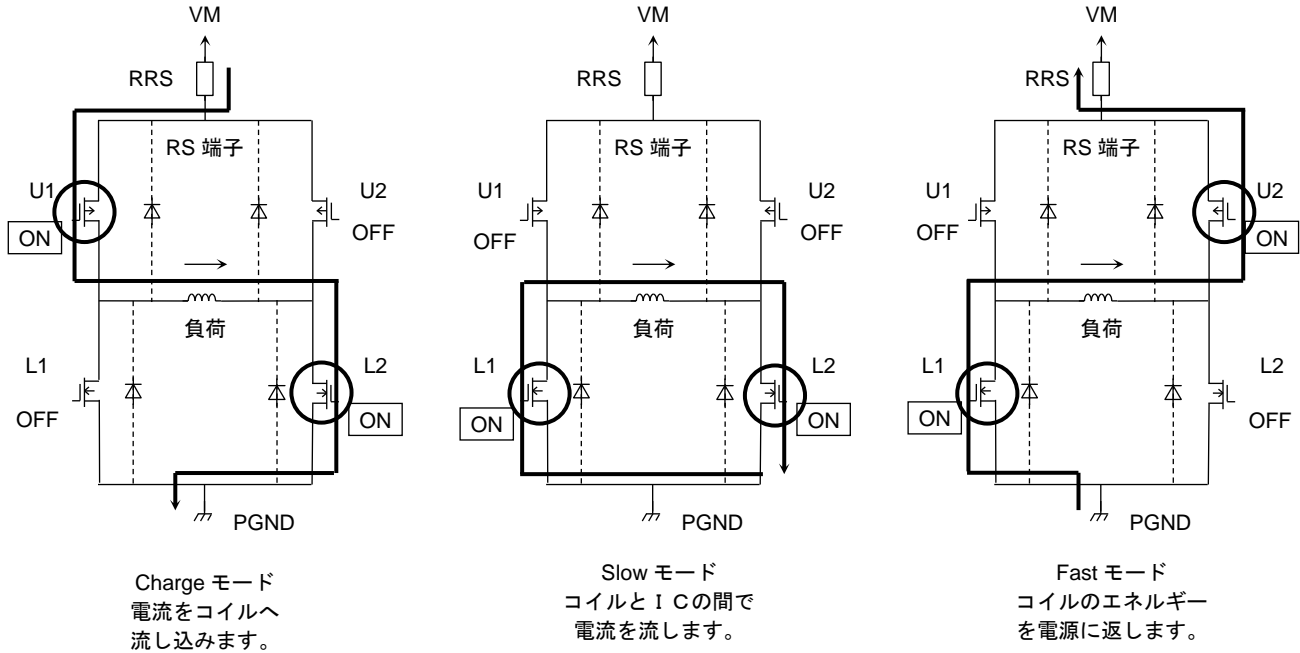
図 6.15 出力段トランジスタ動作モード
