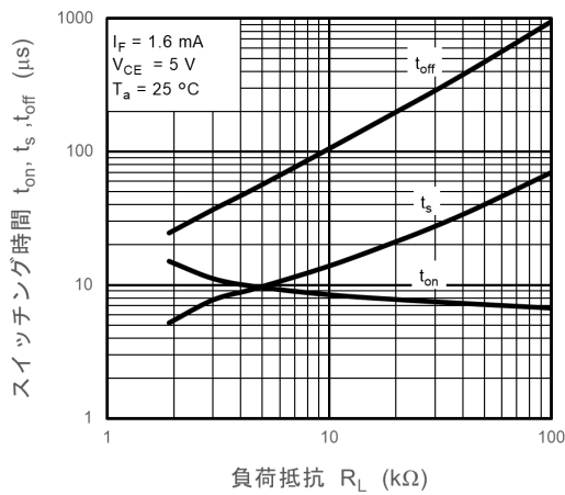
図 12.15 スイッチング時間 - R_L
