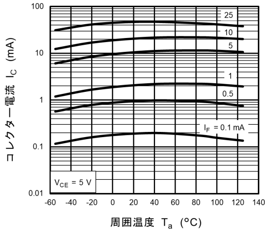
図 12.13 I_C - T_a
