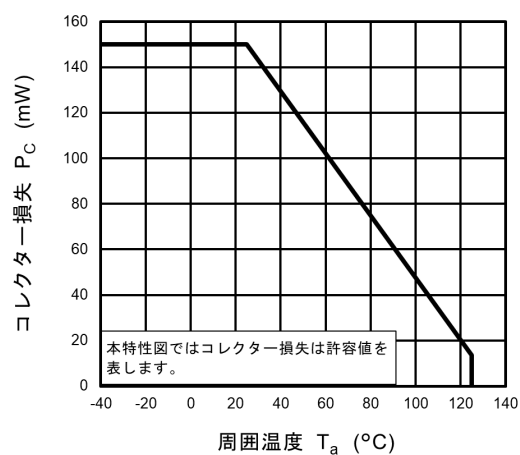
図 12.2 P_C - T_a
