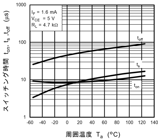
図 12.17 スイッチング時間 - T_a
