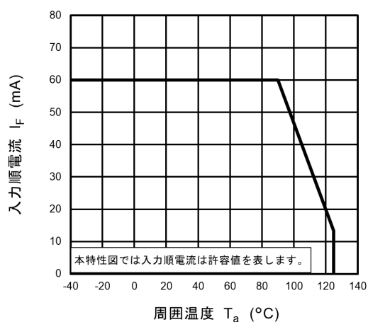
図 12.1 I_F - T_a
