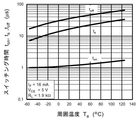
図 12.16 スイッチング時間 - T_a
