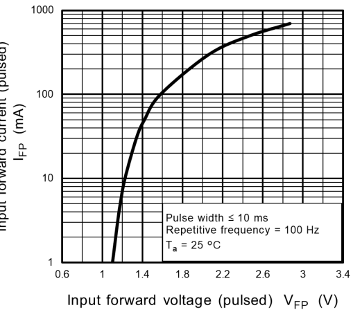
Fig. 12.6 I_{FP} - V_{FP}
