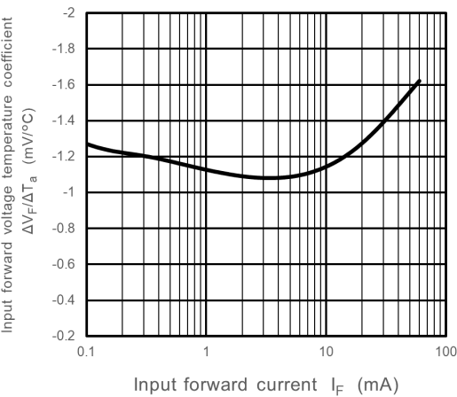
Fig. 12.5 \Delta V_F / \Delta T_a - I_F
