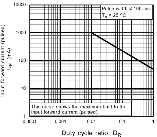
Fig. 12.3 I_{FP} - D_R
