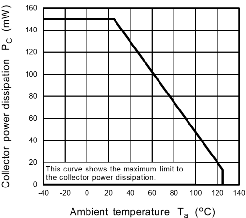
Fig. 12.2 P_C - T_a
