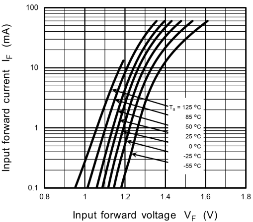
Fig. 12.4 I_F - V_F
