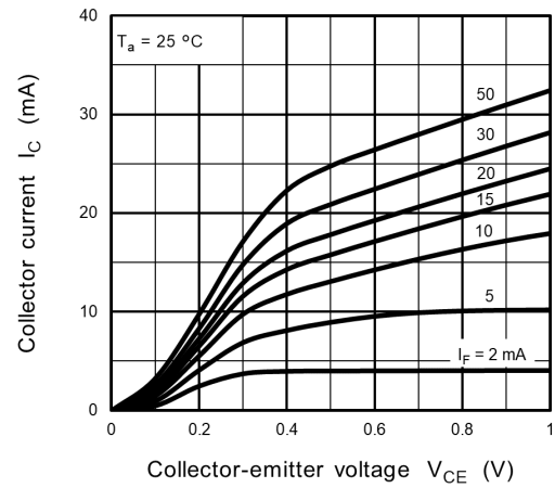
Fig. 12.8 I_C - V_{CE}
