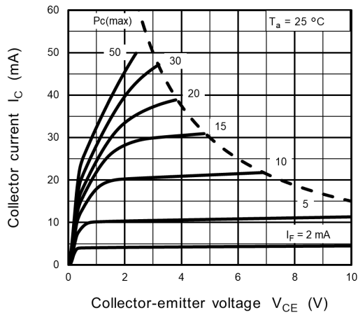
Fig. 12.7 I_C - V_{CE}
