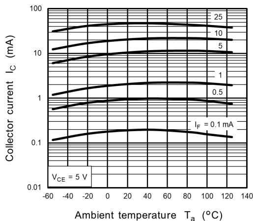
Fig. 12.13 I_C - T_a
