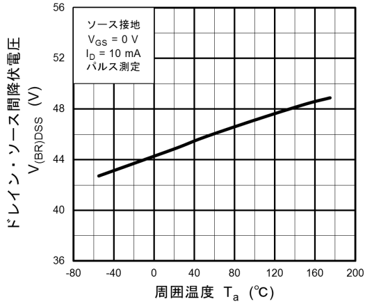
図 8.7 V_{(BR)DSS} - T_a
