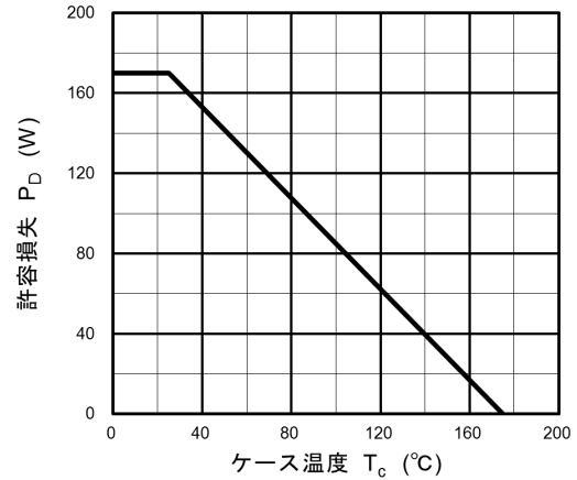
図 8.15 P_D - T_c (最大値 (保証値))
