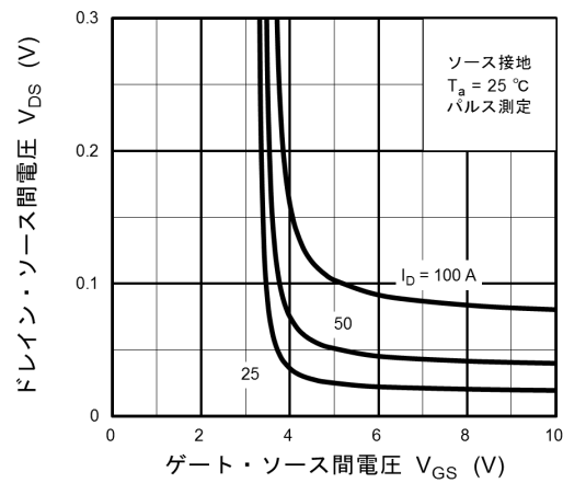
図 8.4 V_{DS} - V_{GS}
