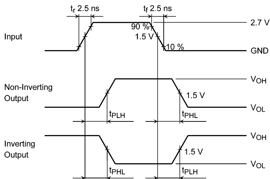
図 12.8.1 t_{PLH} , t_{PHL}
