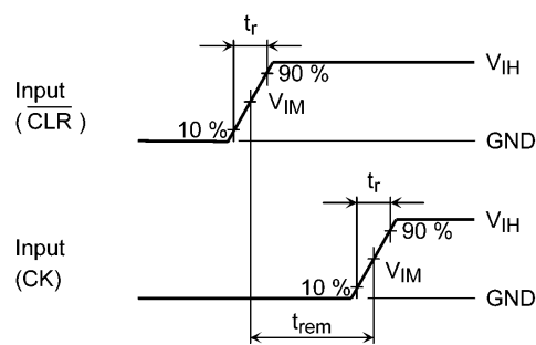
図 12.8.3 t_{rem}
