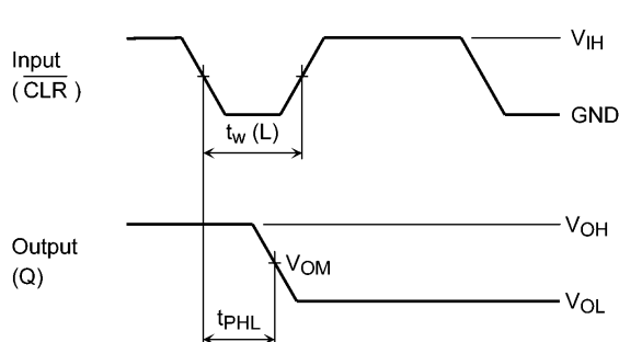
図 12.8.2 t_{PHL} , t_w
