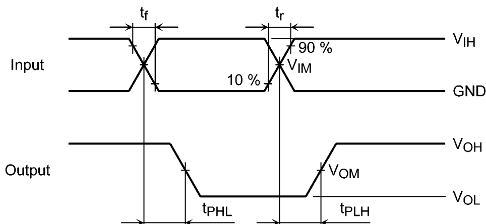
図 11.8.1 t_{PLH} , t_{PHL}
