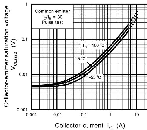
Fig. 7.4 V_{CE(sat)} - I_C
