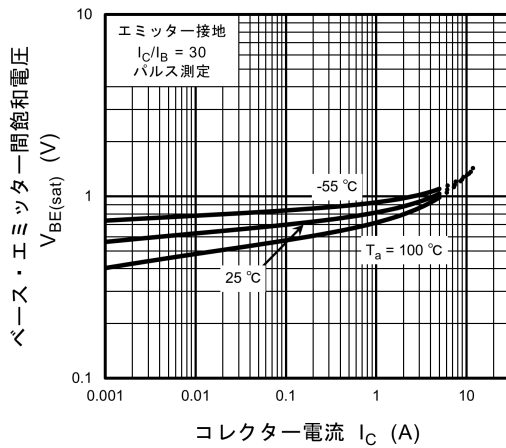
図 7.5 V_{BE(sat)} - I_C
