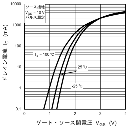
図 8.3 I_D - V_{GS}
