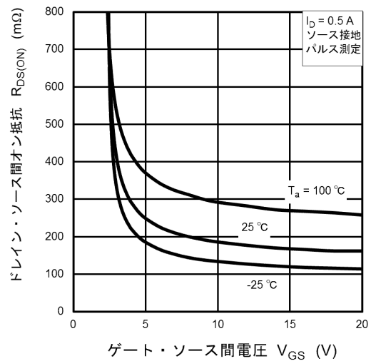
図 8.4 R_{DS(ON)} - V_{GS}
