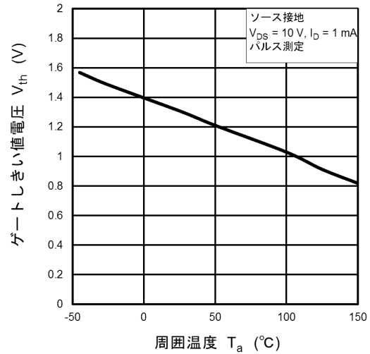
図 8.8 V_{th} - T_a
