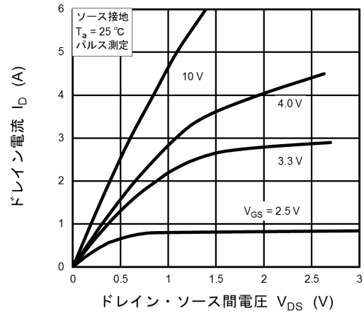
図 8.2 I_D - V_{DS}
