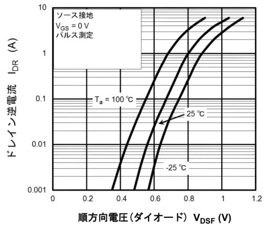
図 8.10 I_{DR} - V_{DSF}
