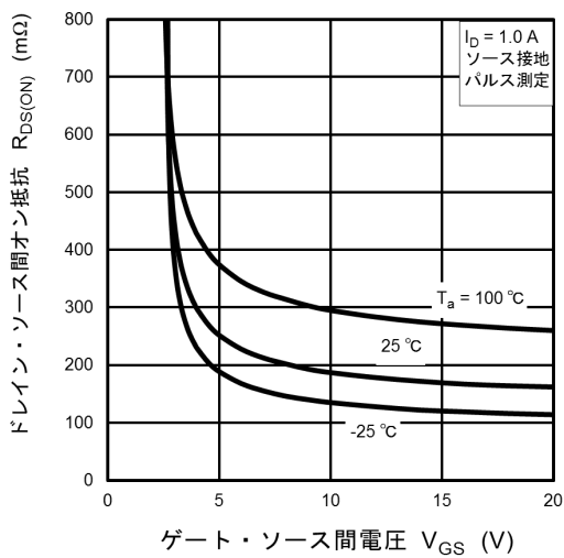
図 8.5 R_{DS(ON)} - V_{GS}
