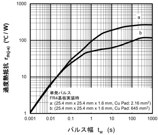
図 8.13 r_{th(j-a)} - t_w
