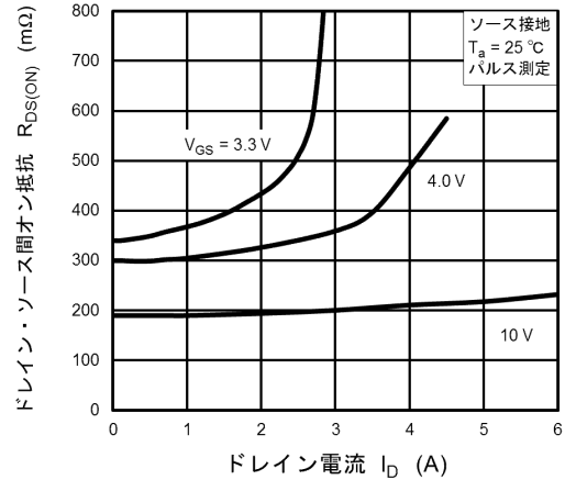
図 8.6 R_{DS(ON)} - I_D
