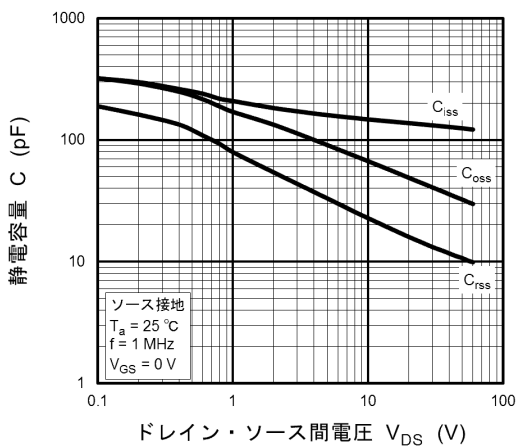
図 8.11 C - V_{DS}
