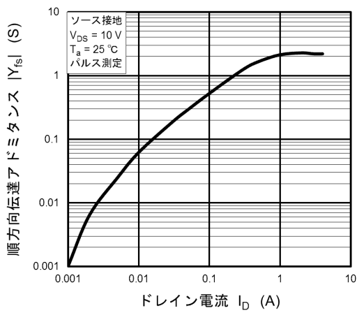
図 8.9 |Y_{fs}| - I_D
