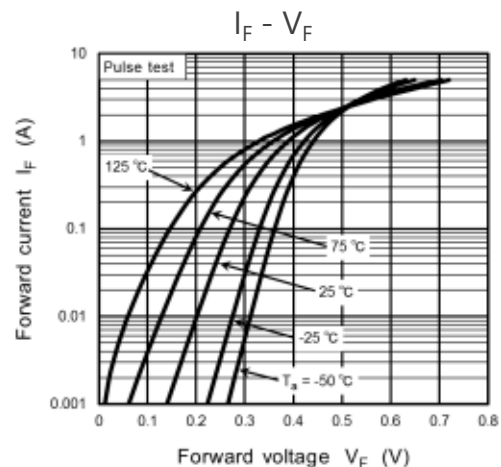
CUHS20F40特性図
