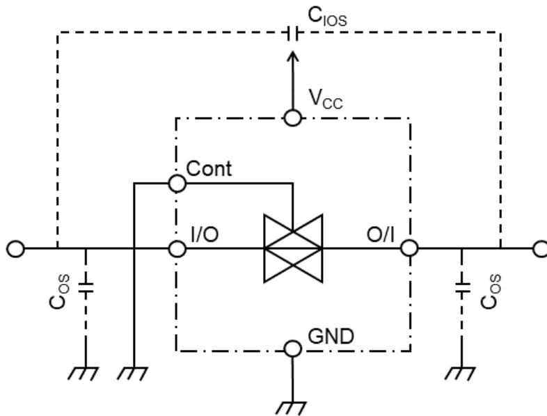
図 2 C ios , C os
