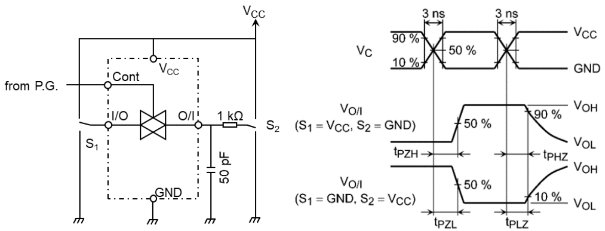
図 1 t PLZ , t PHZ , t PZL , t PZH
