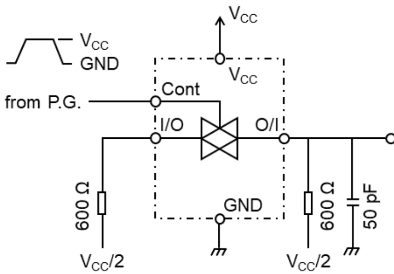
図 5 クロストーク (コントロール入カスイッチ出力)
