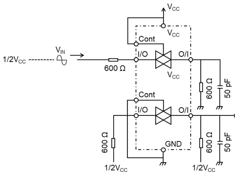
図 6 クロストーク (スイッチ間)
