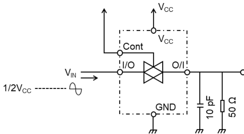
図 3 最大伝達周波数
