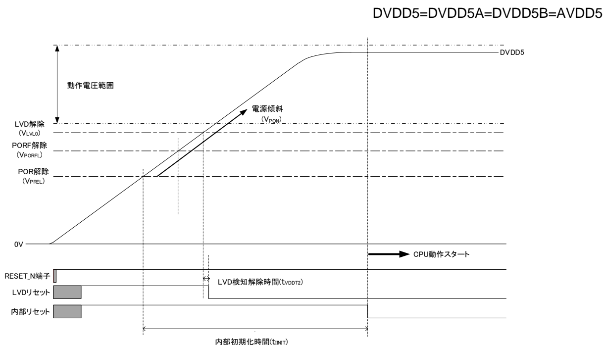
図 3.1 パワーオンリセット回路によるリセット動作
