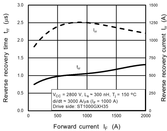
Fig. 7.11 t_{rr} , I_{rr} - I_F
