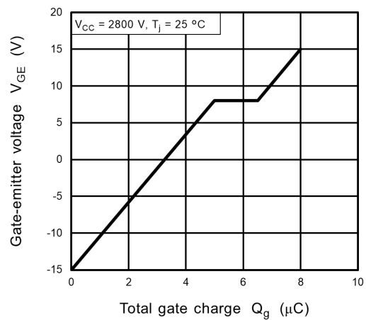
Fig. 7.12 V_{GE} - Q_g
