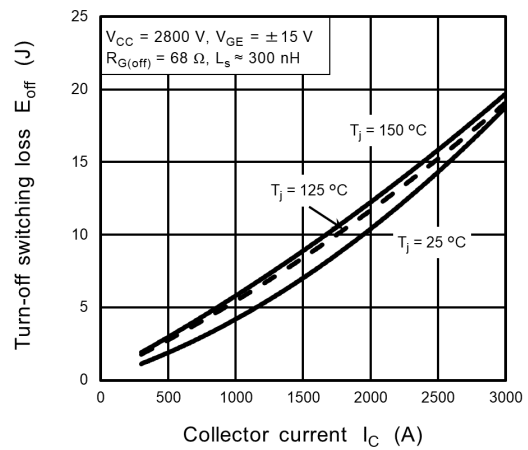
Fig. 7.6 E_{off} - I_C
