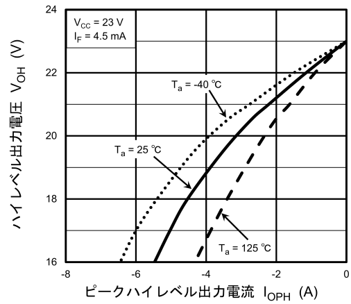
図 13.2.10 (V_{OH} - V_{CC}) - I_{OPH}
