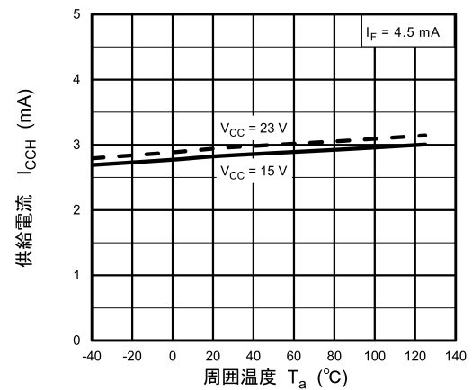
図 13.2.6 I_{CCH} - T_a
