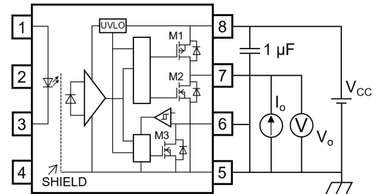
图 13.1.4 V_{OL} 测定回路
