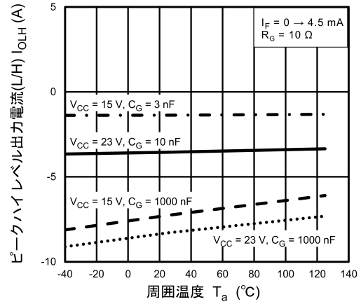
図 13.2.14 I_{OLH} - T_a
