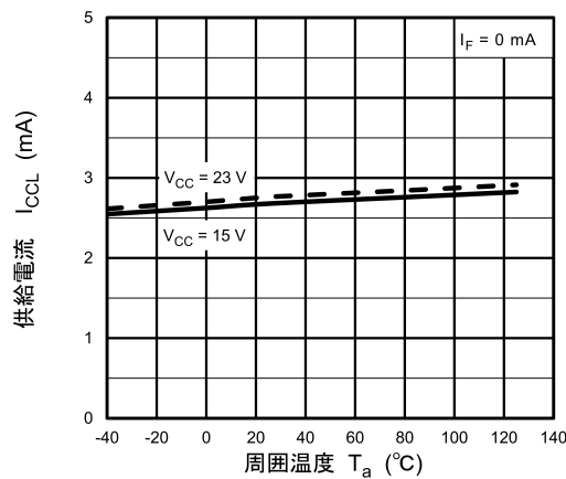
図 13.2.5 I_{CCL} - T_a
