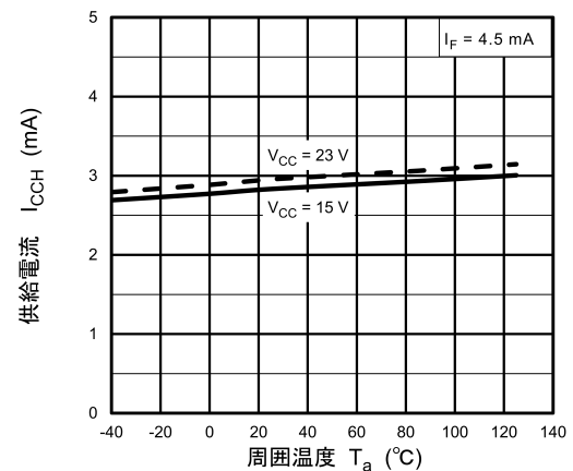
図 13.2.6 I_{CCH} - T_a
