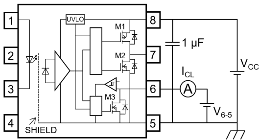
图 13.1.5 I_{CLAMP} 测定回路
