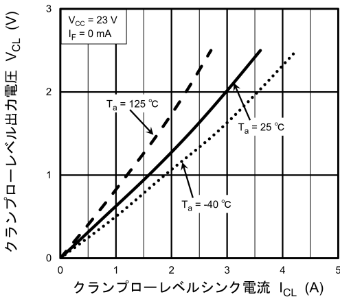
図 13.2.11 V_{CLAMP} - I_{CLAMP}
