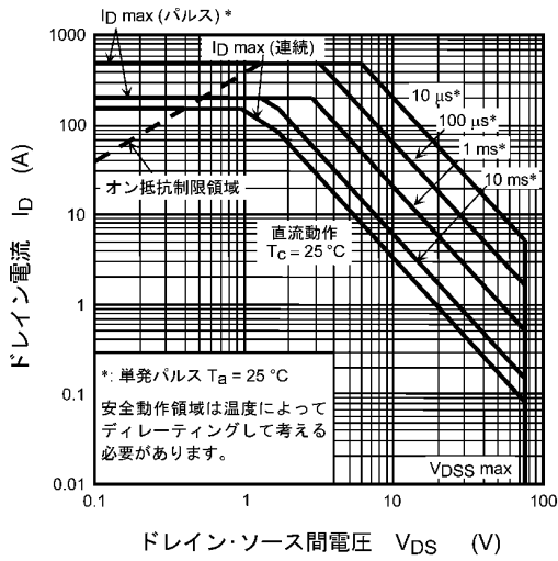
ドレイン・ソース間電圧 V_{DS} (V) 図 8.14 安全動作領域 (最大値 (保証値))
