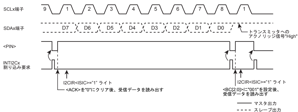
図 13-13 マスタレシーバモード時、データの送信を終了させるときの処理
