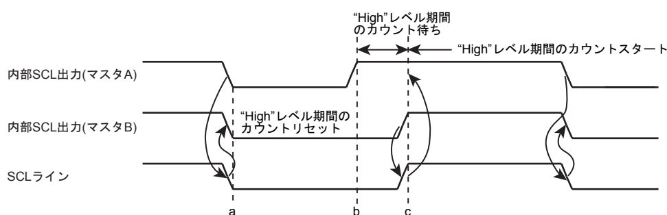
図 13-5 クロック同期化の例
