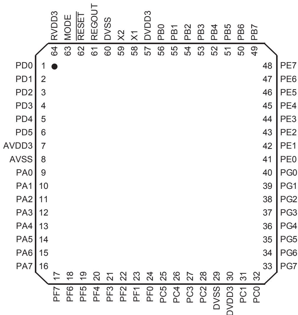
図 1-2 ピン配置図(LQFP64 TOP VIEW)
