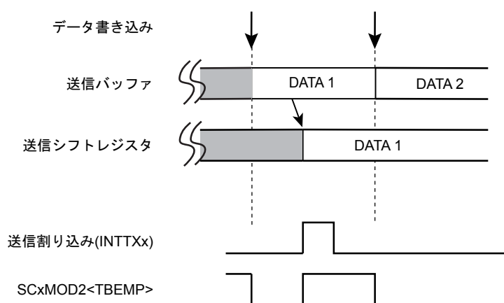
図 12-8 送信バッファの動作(ダブルバッファ有効時)
