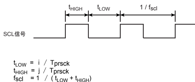
図 13-4 クロックソース
