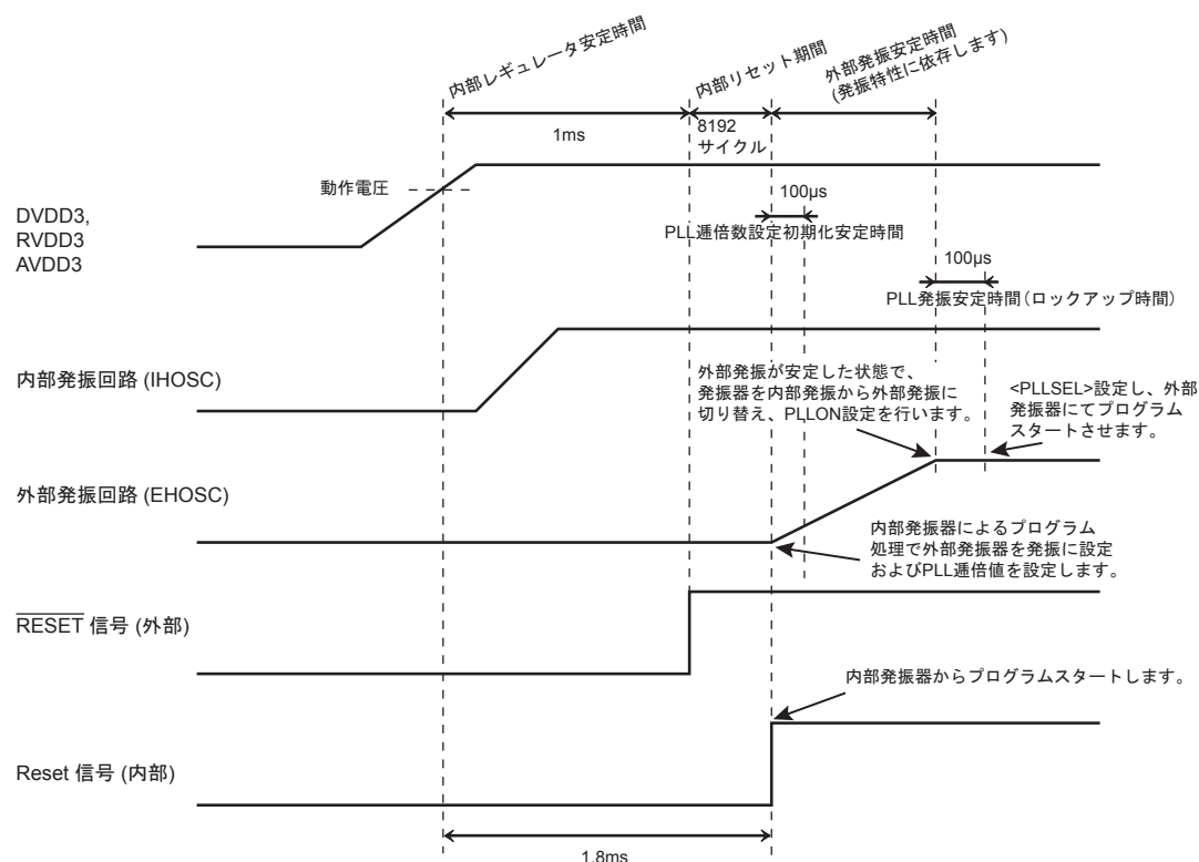
図 6-2 外部高速発振器を使用し PLL 通倍回路を設定した場合の遷移
