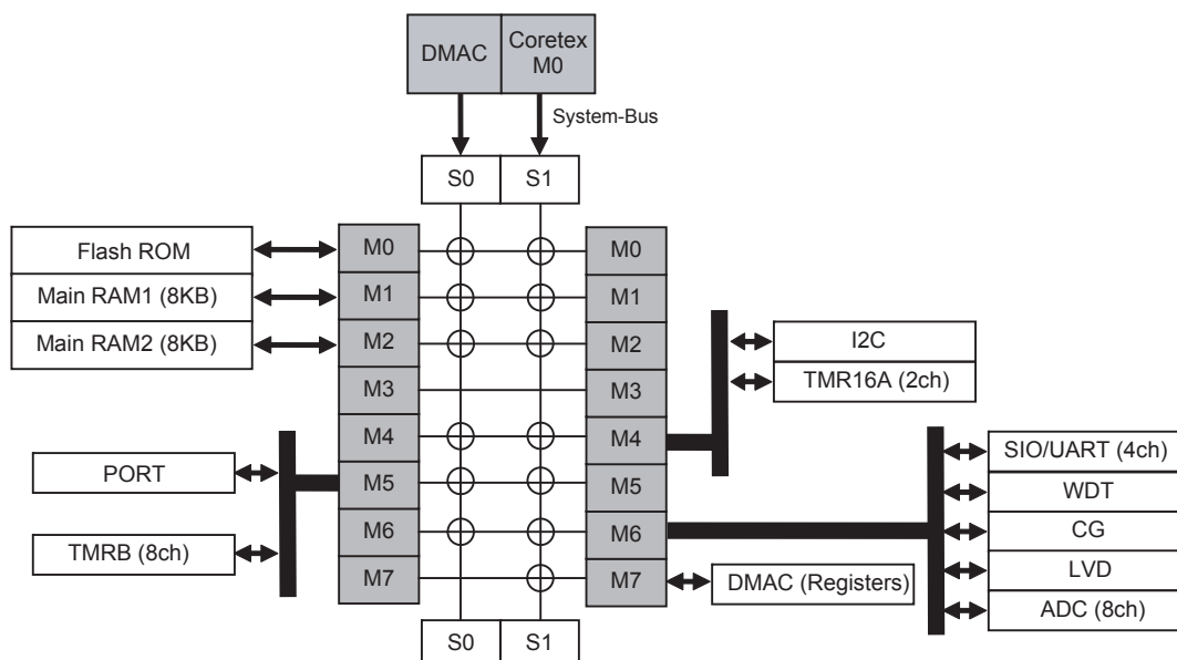
図 4-2 TMPM037FWUG (シングルチップモード)
