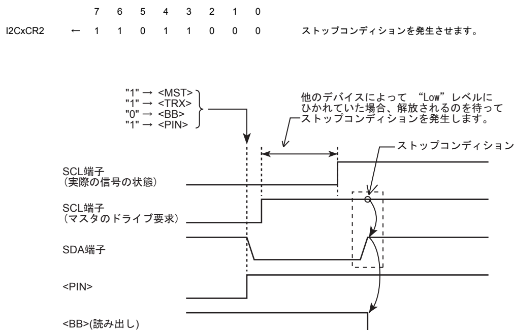
図 13-14 ストップコンディションの発生
