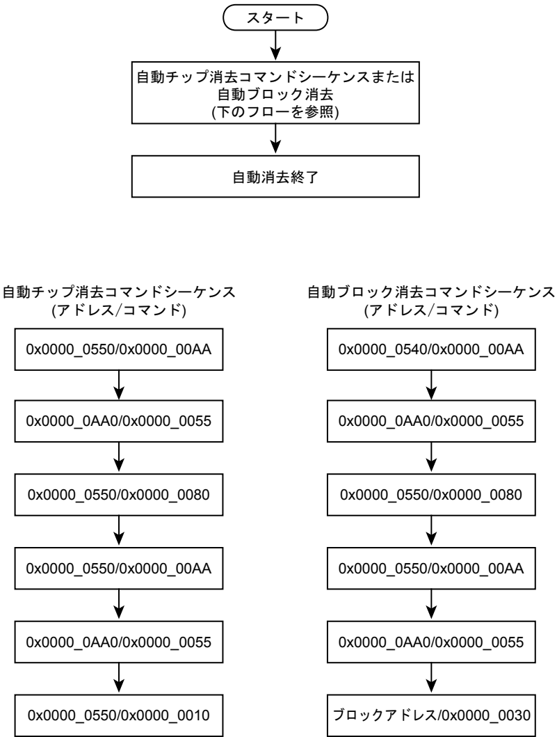
図 17-5 自動消去フローチャート
