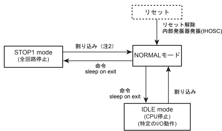
図 6-3 モード状態遷移図
