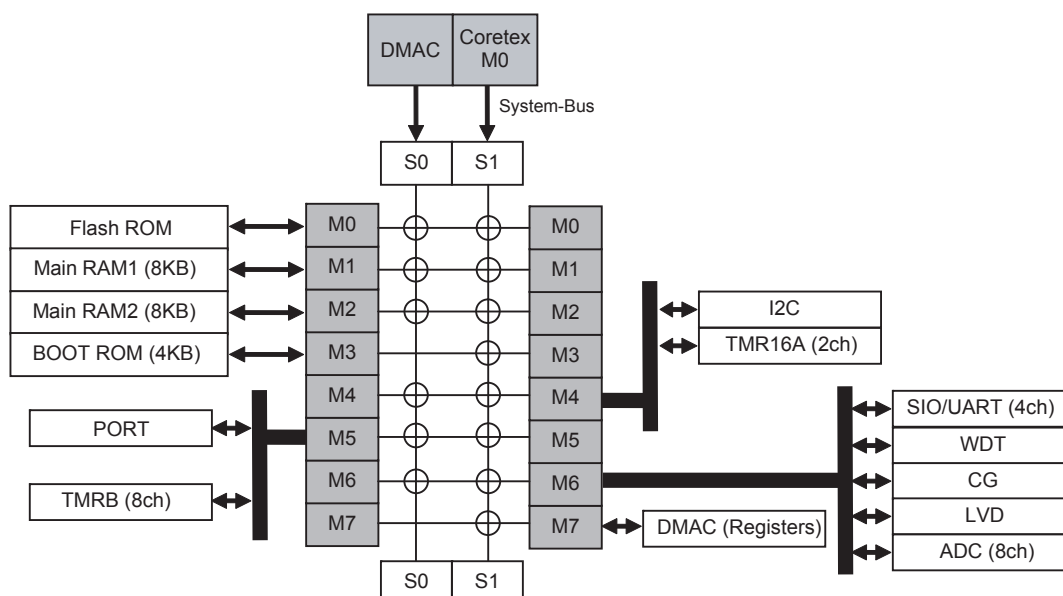
図 4-3 TMPM037FWUG (シングルブートモード)
