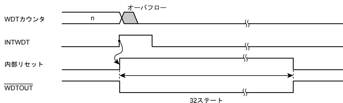
図 16-3 内部リセット発生
