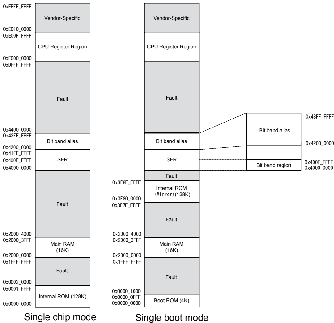
図 4-1 TMPM037FWUG メモリマップ
