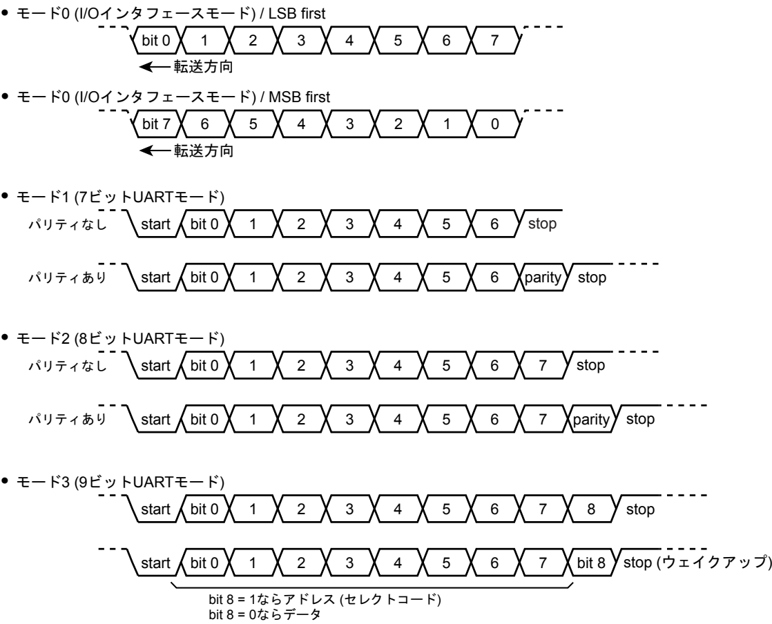
図 12-3 データフォーマット
