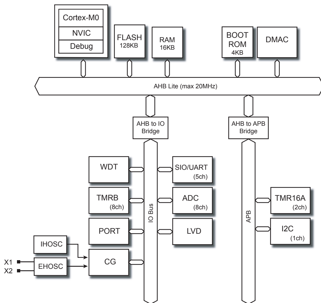
図 1-1 ブロック図
