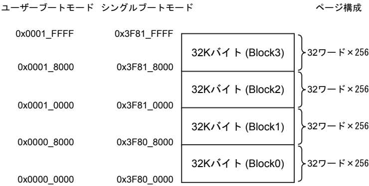
図 17-1 ブロック構成
