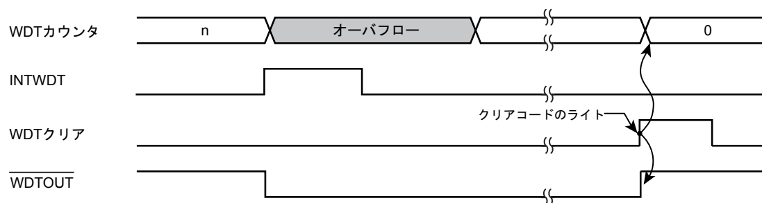
図 16-2 INTWDT 割り込み発生
