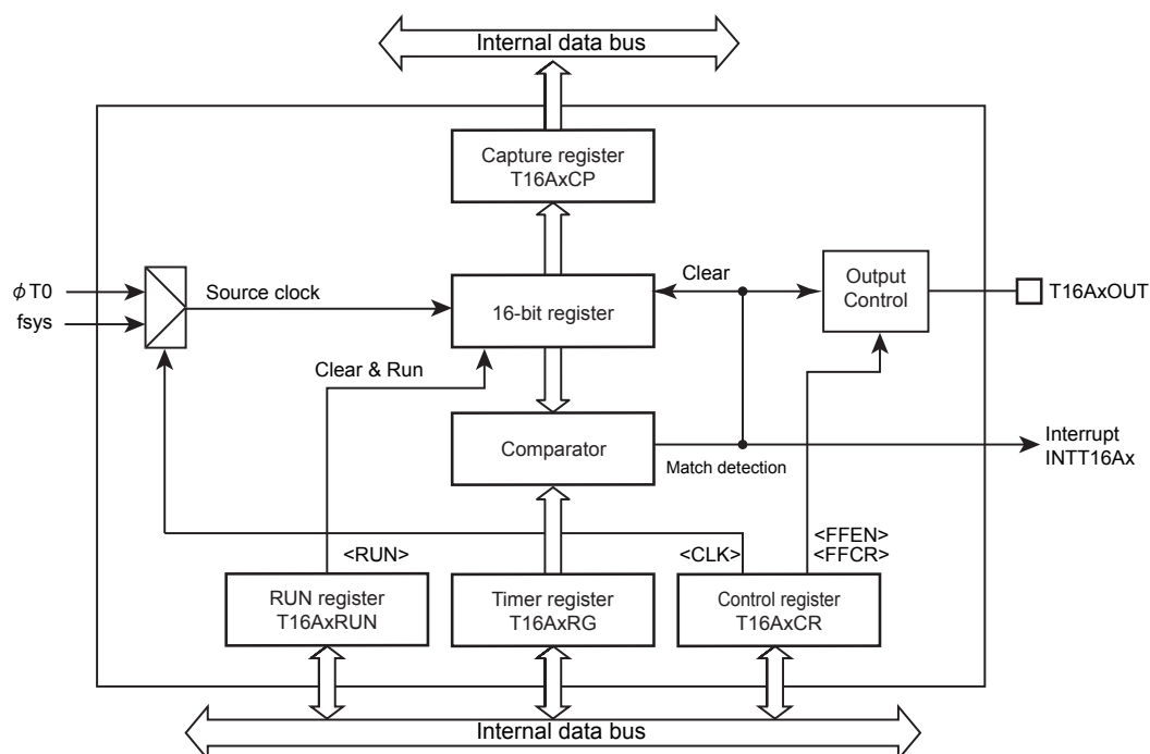
図 11-1 TMR16Ax ブロック図
