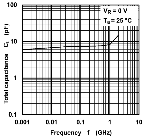
図 7.4 C_t - f
