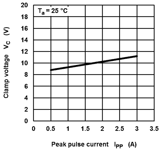
図 8.1 V_C - I_{PP}
