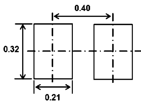
図 6.1 参考Pad寸法 (Unit: mm)
