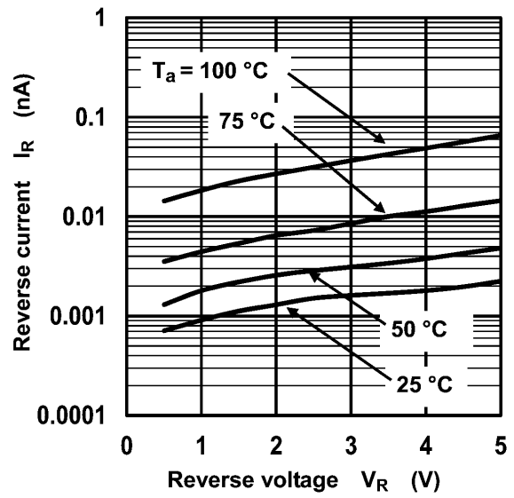
図 7.2 I_R - V_R
