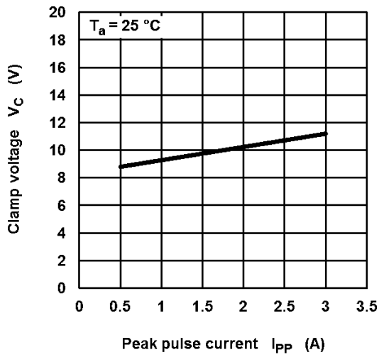
図 8.1 V_C - I_{PP}
