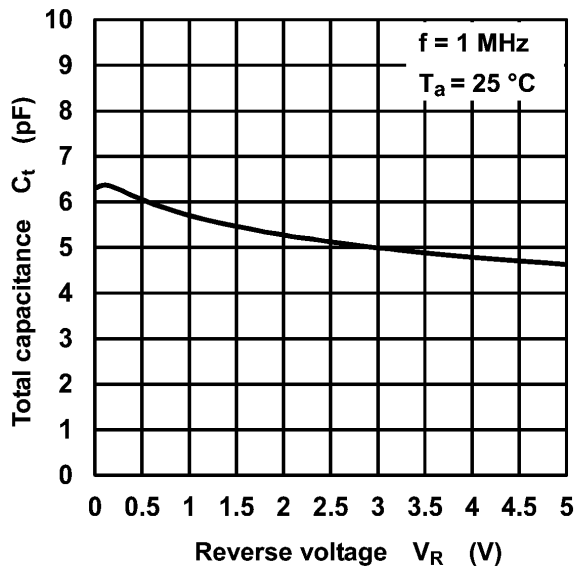
図 7.3 C_t - V_R
