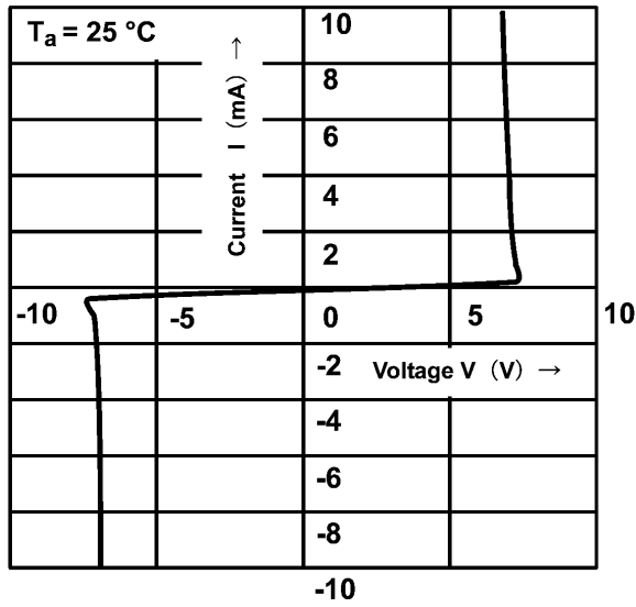
図 7.1 I - V
