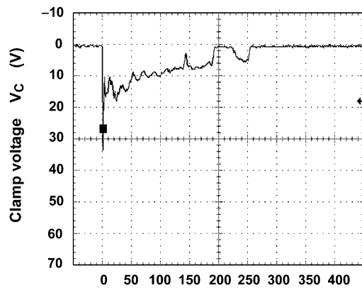
Pulse time t_p (ns) 図 10.2 -8 kV
