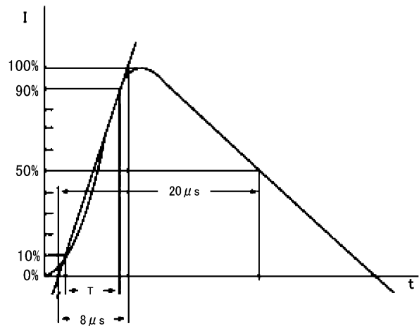
図 8.2 IEC61000-4-5準拠 8/20 \mu s
