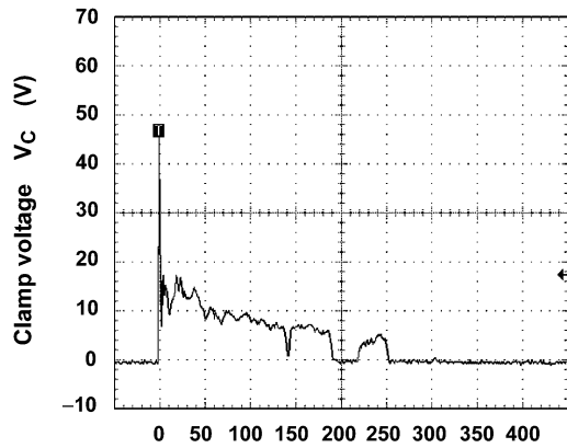
Pulse time t_p (ns) 図 10.1 +8 kV
