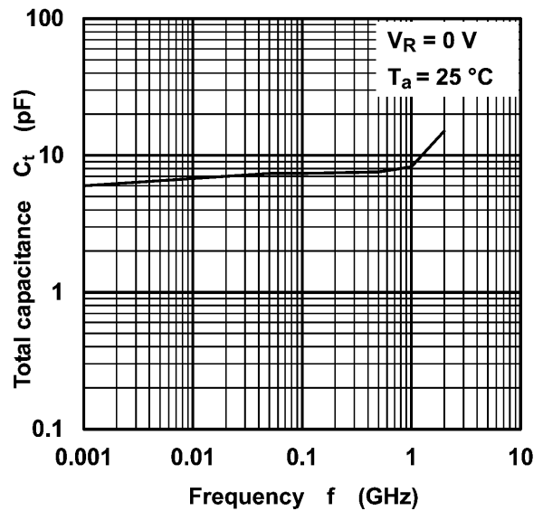
図 7.4 C_t - f
