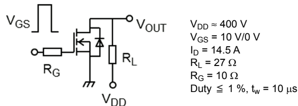
図 6.2.1 スイッチング時間の測定回路
