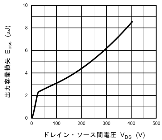
図 8.12 E oss - V DS
